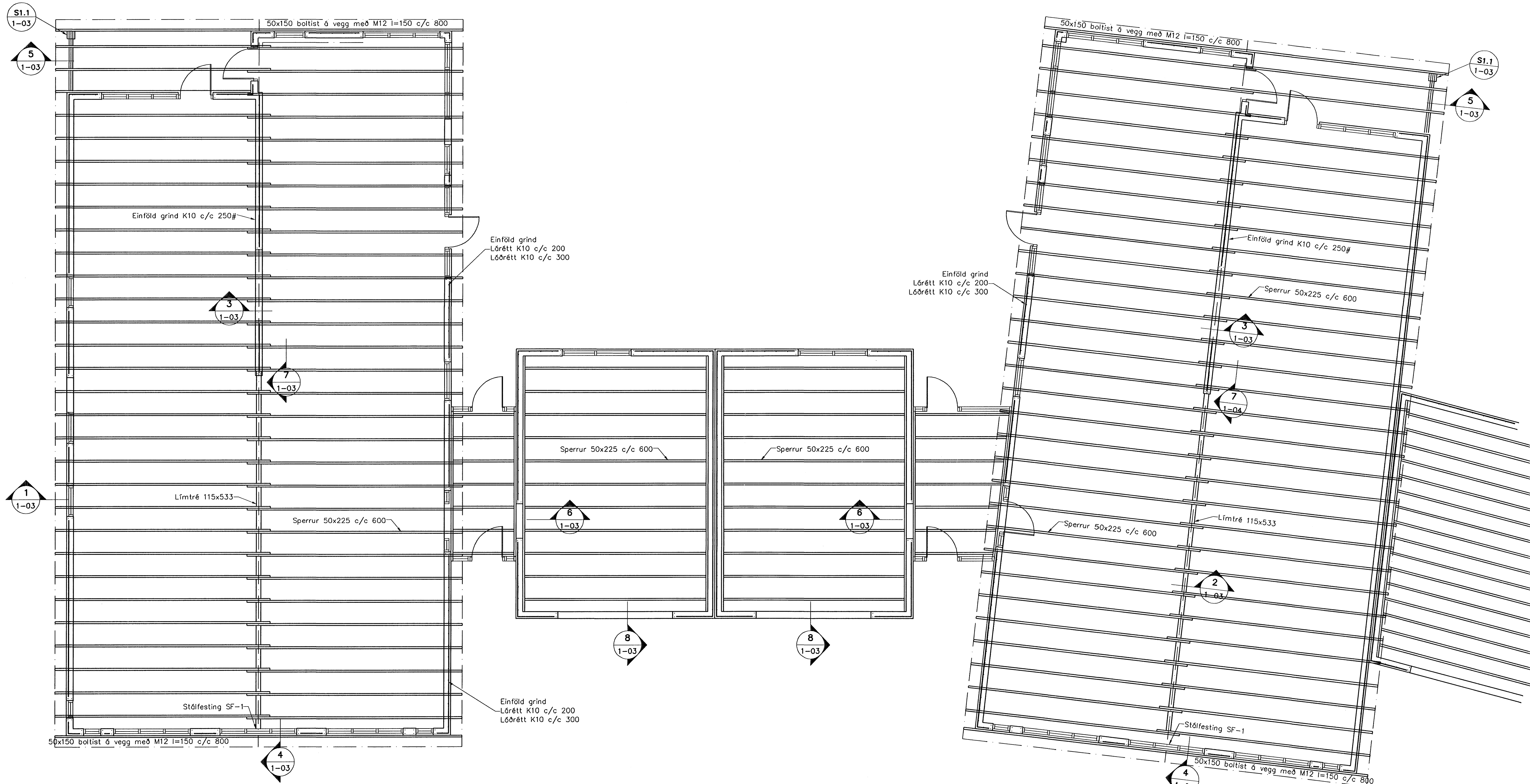
Veggir, Þakvirki, Grunnmynd, 1:50
