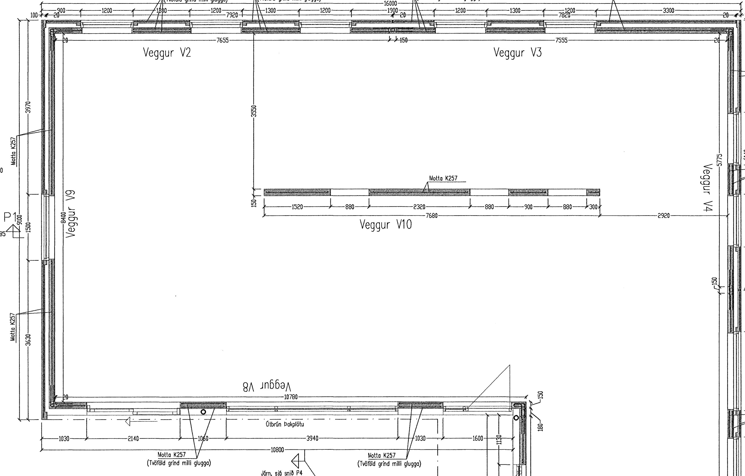
Grunnmynd burðarveggja 1:50
