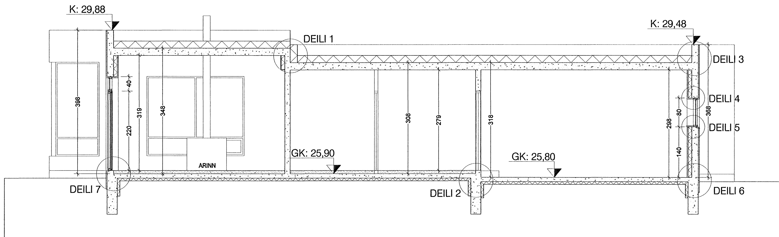
SNEIÐING A-A
