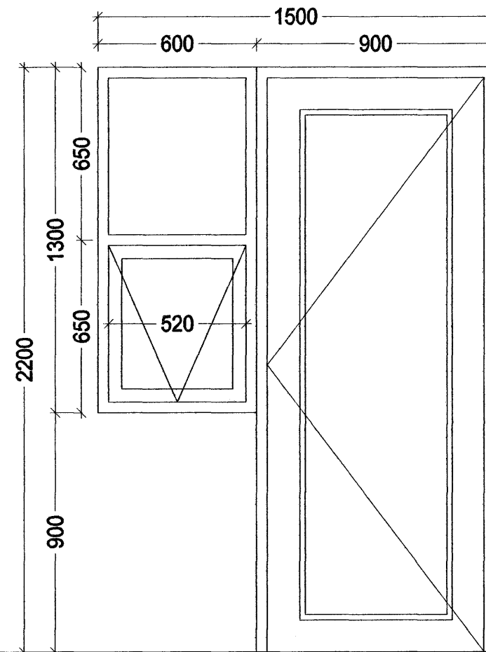
H3 1.stk Hægri út
