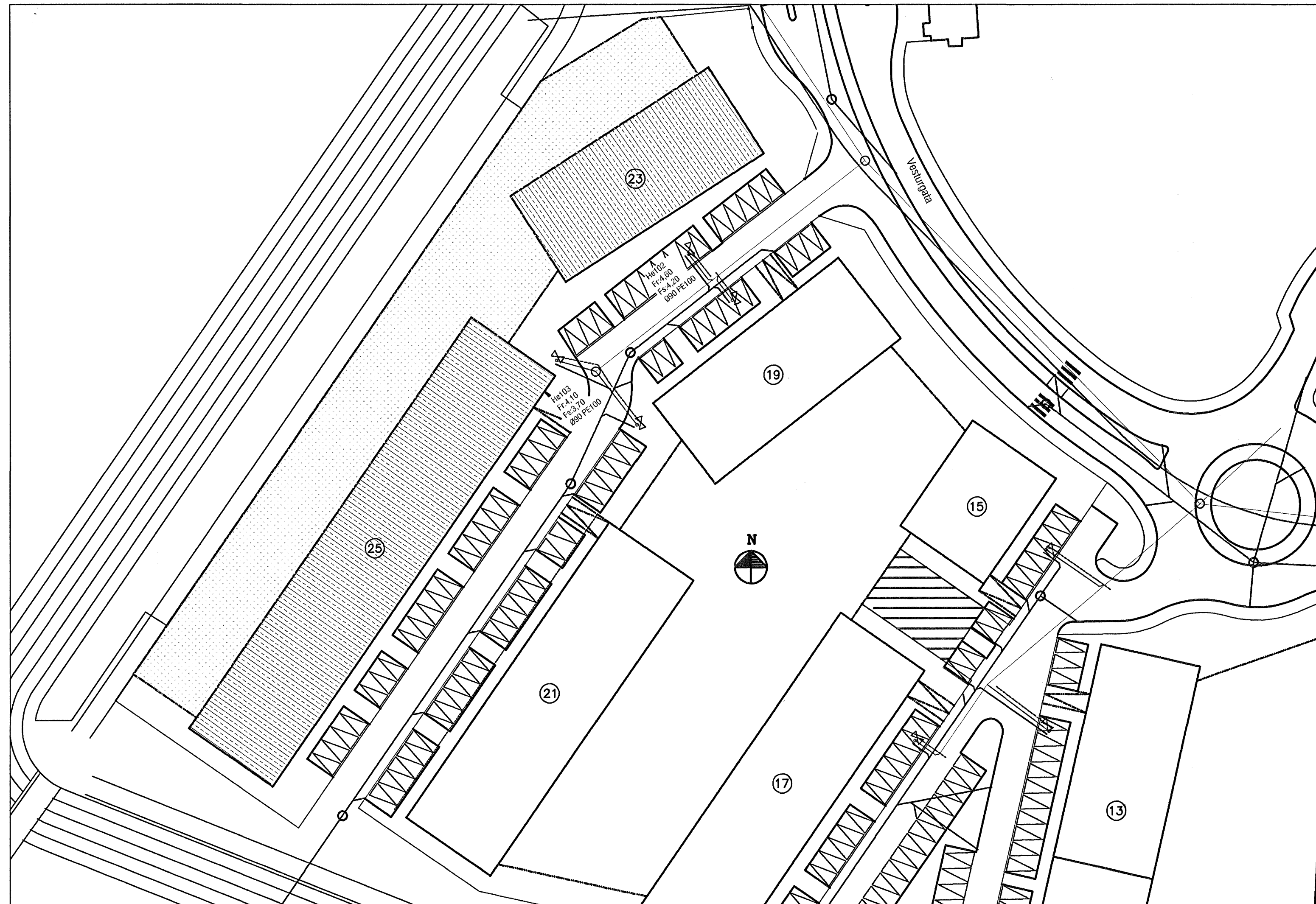
AFSTÖÐUMYND 1:500
