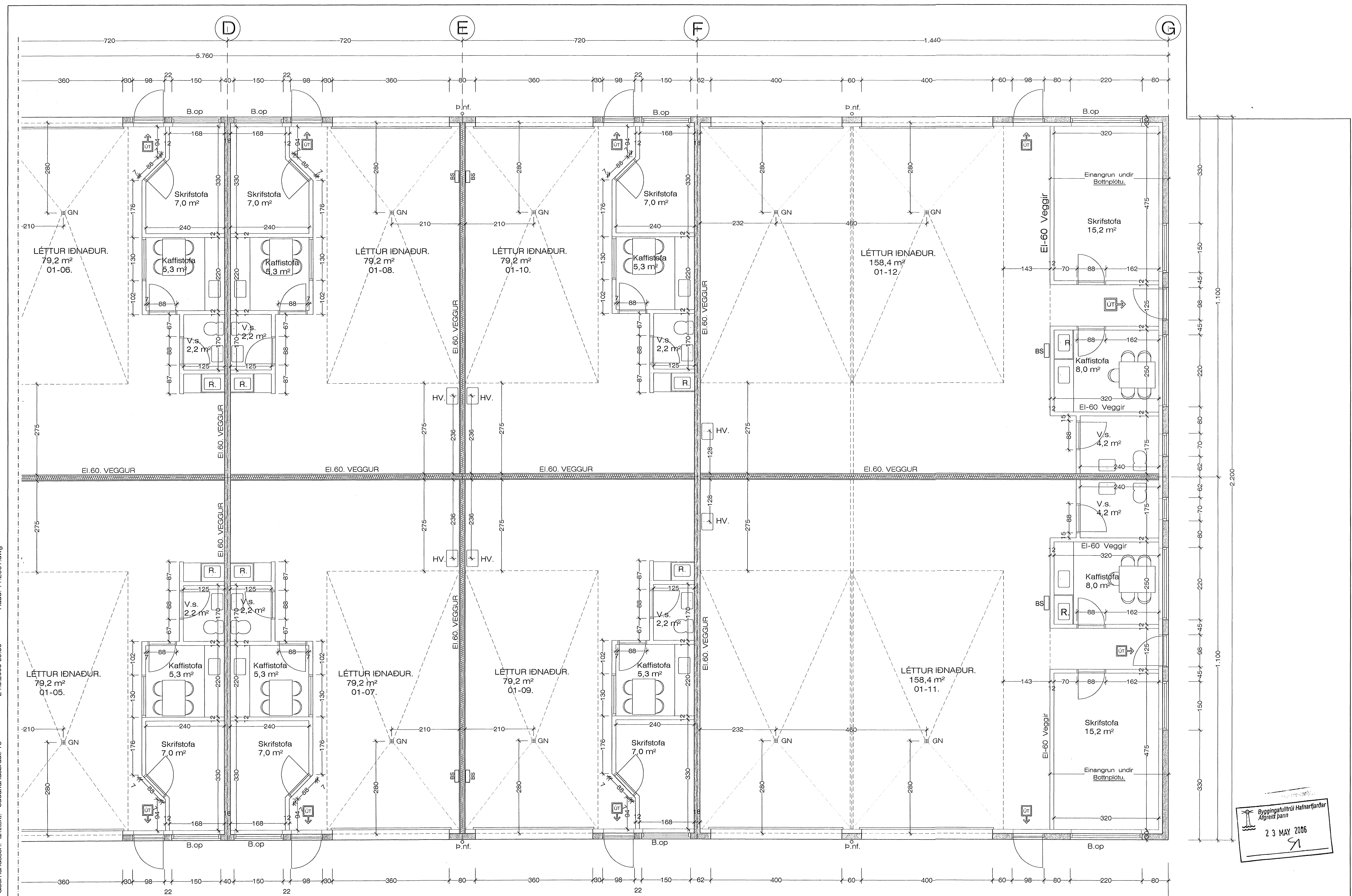
GRUNNMYND JARÐHÆÐAR. B 1:50
