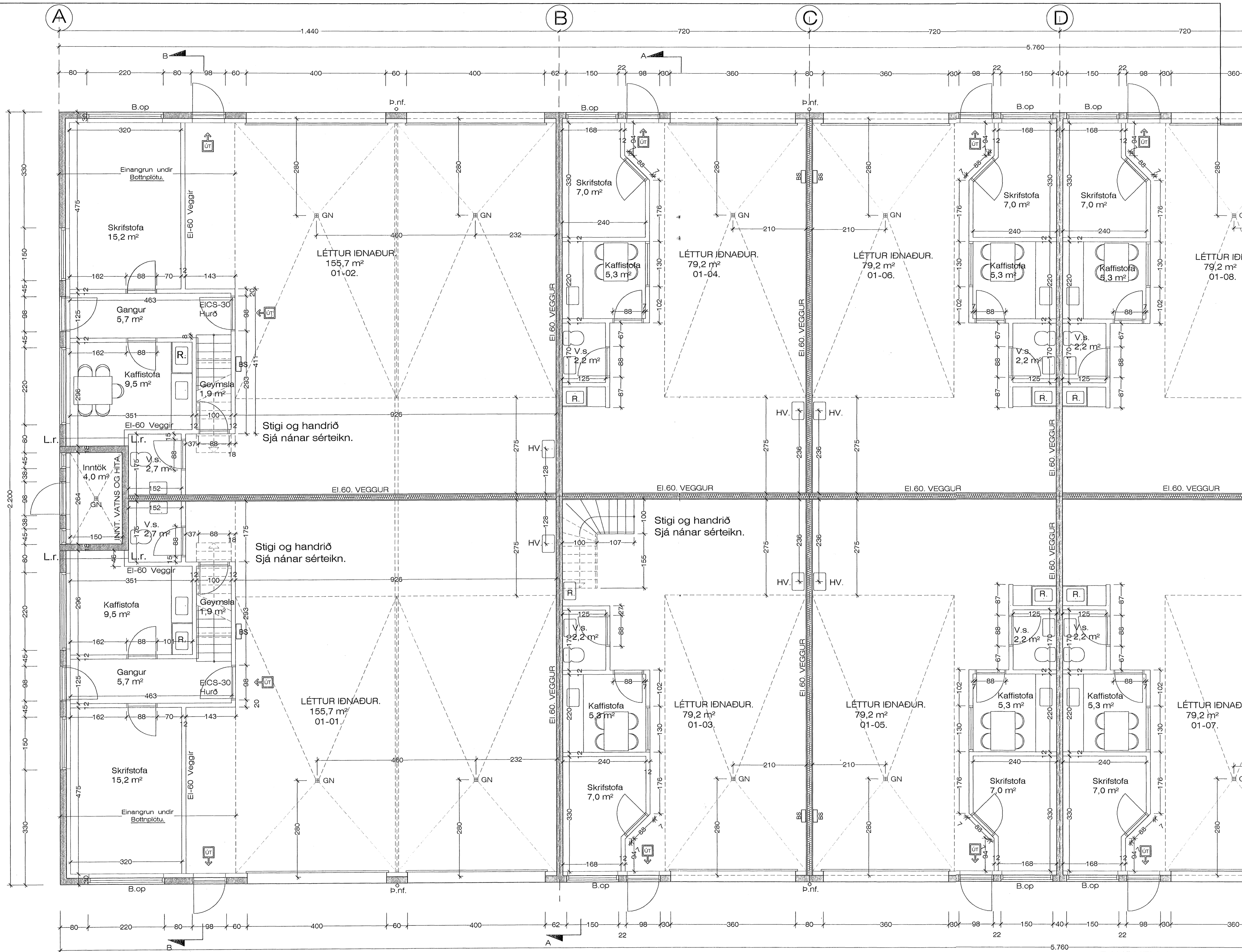
GRUNNMYND JARÐHÆÐAR. A 1:50
