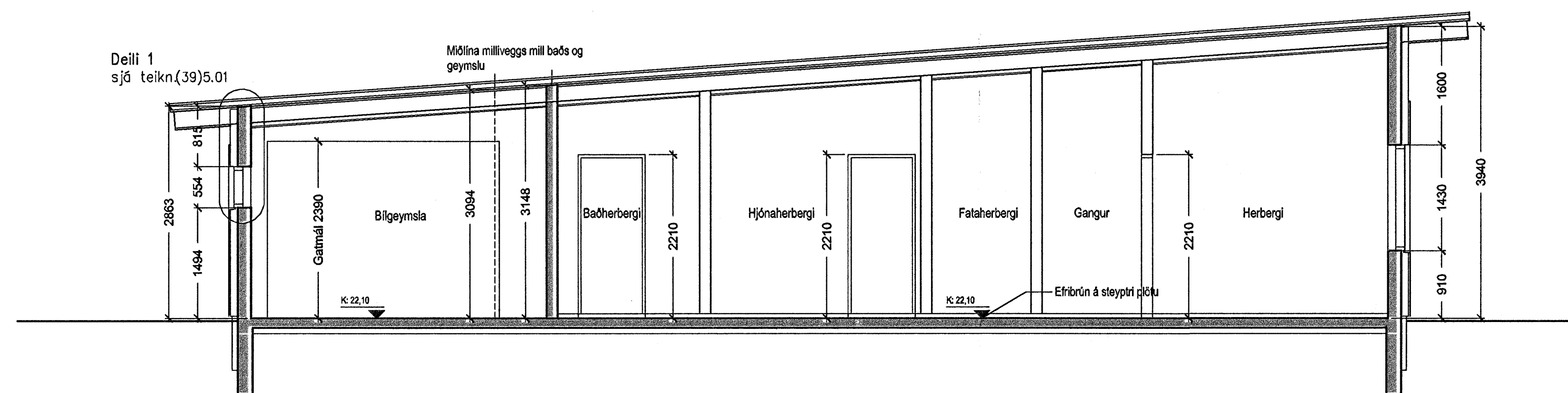
Snið A-A mkv. 1:50
