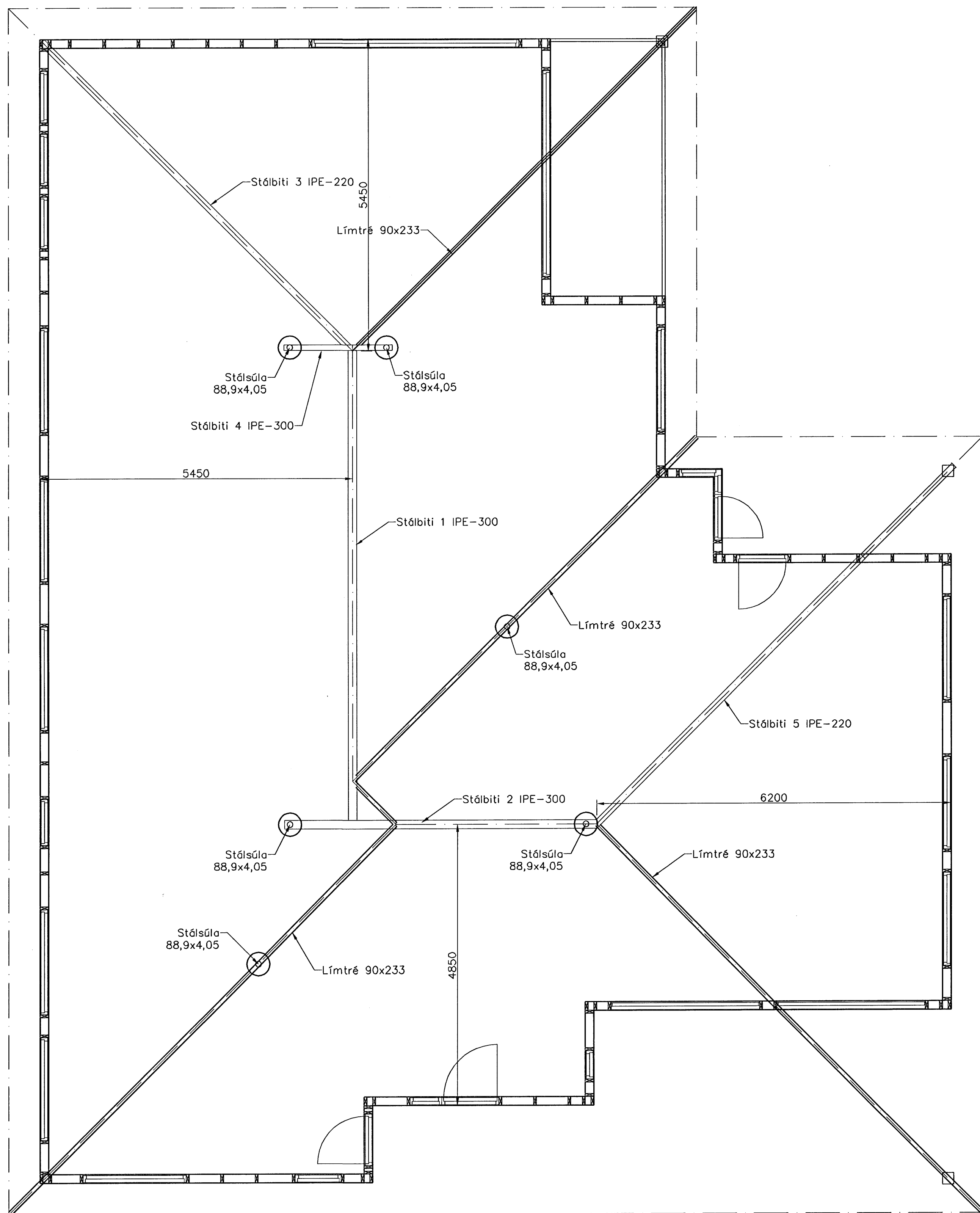
Grunnmynd, 1:50
