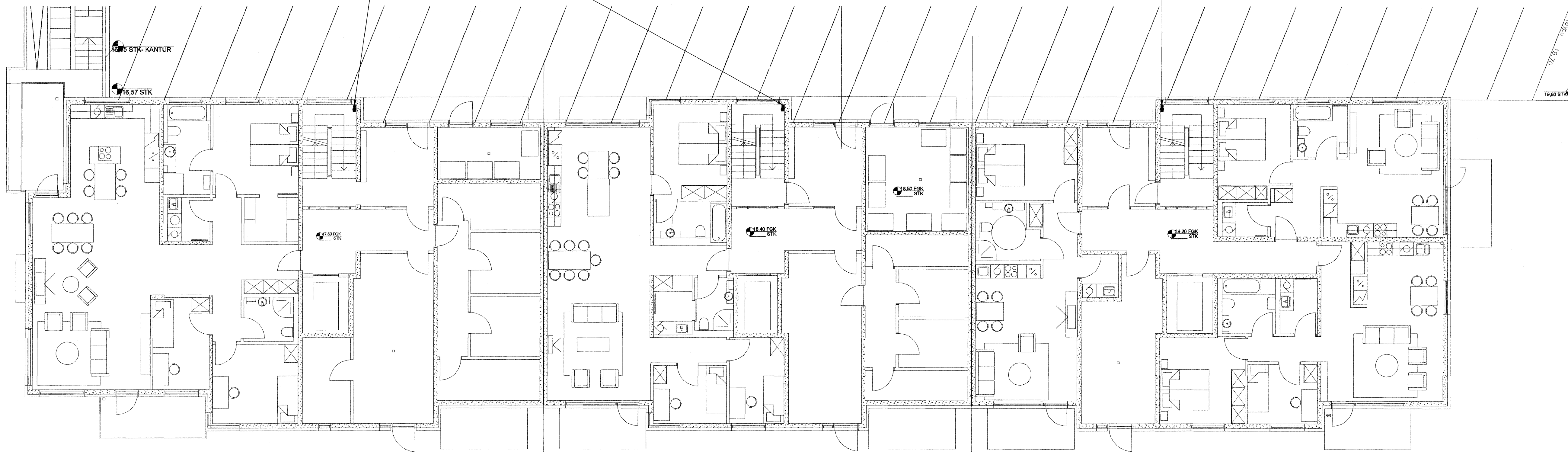
GRUNNMYND 1:100
