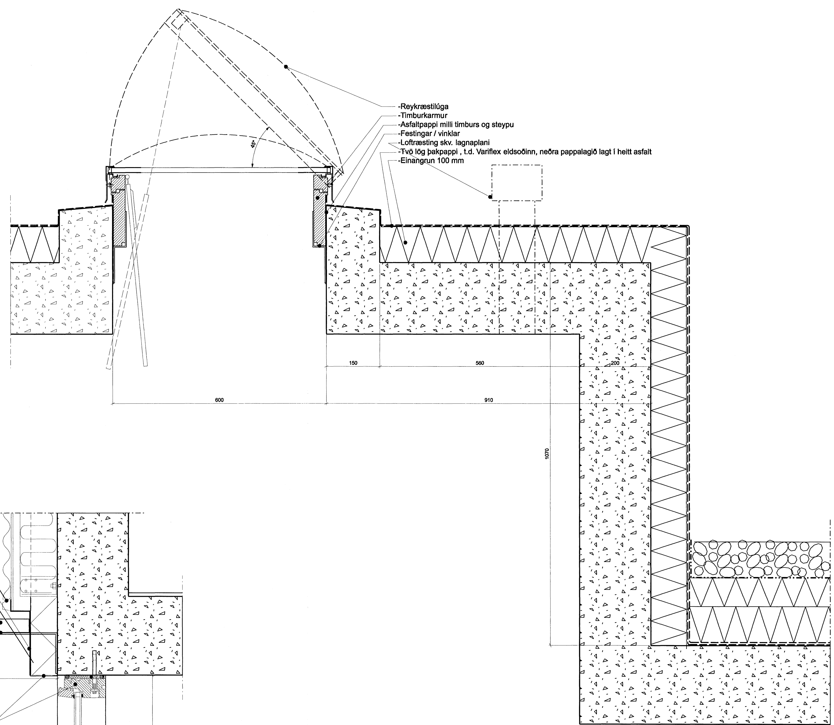
1 DEILI 1:5 Reykræstilúga ofan á lyftuturni
