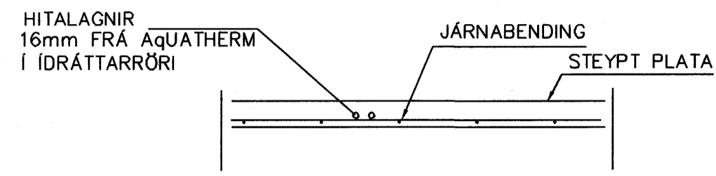
LAGNIR, SNIÐ, 1:20
