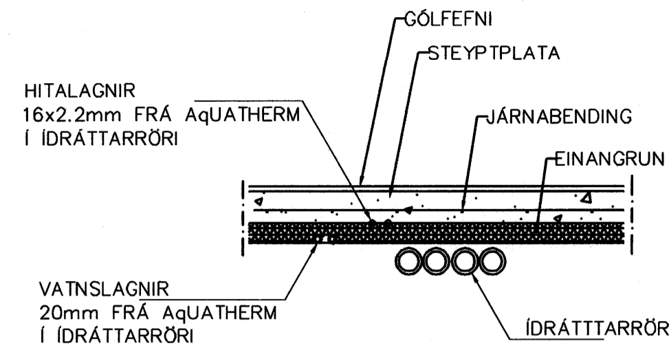
LAGNIR, SNIÐ, 1:20
