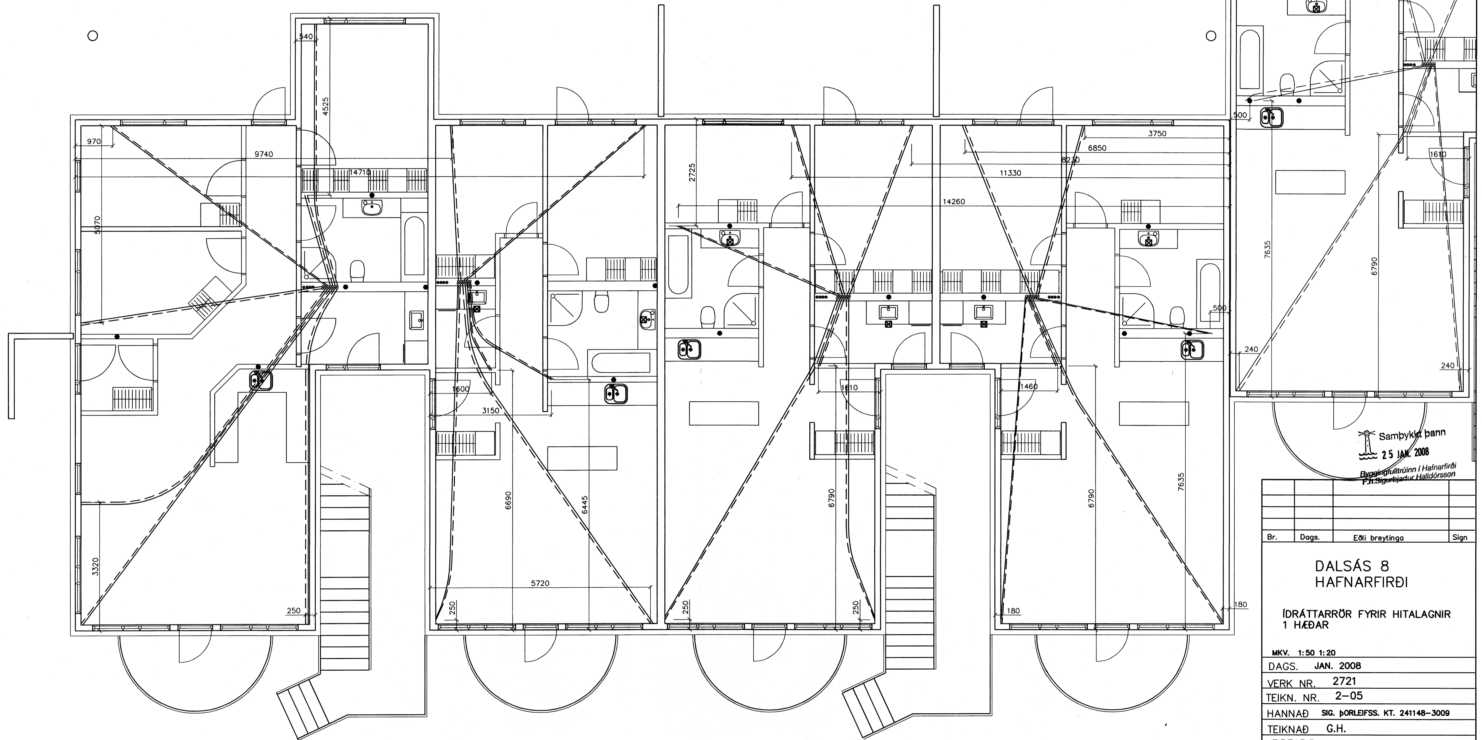
GRUNNMYND 1 HÆÐAR 1:50
