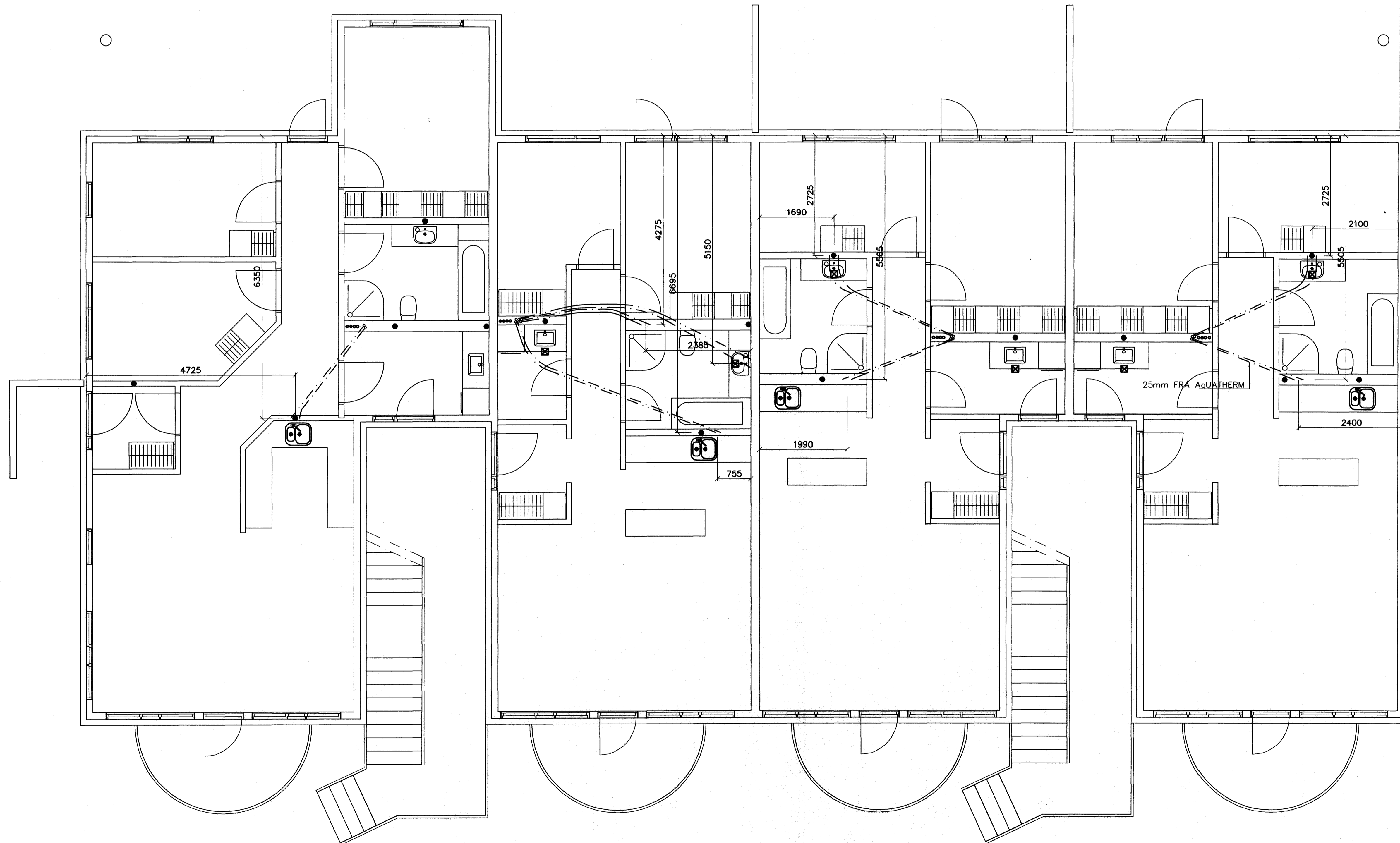
GRUNNMYND 1 HÆÐAR 1:50
