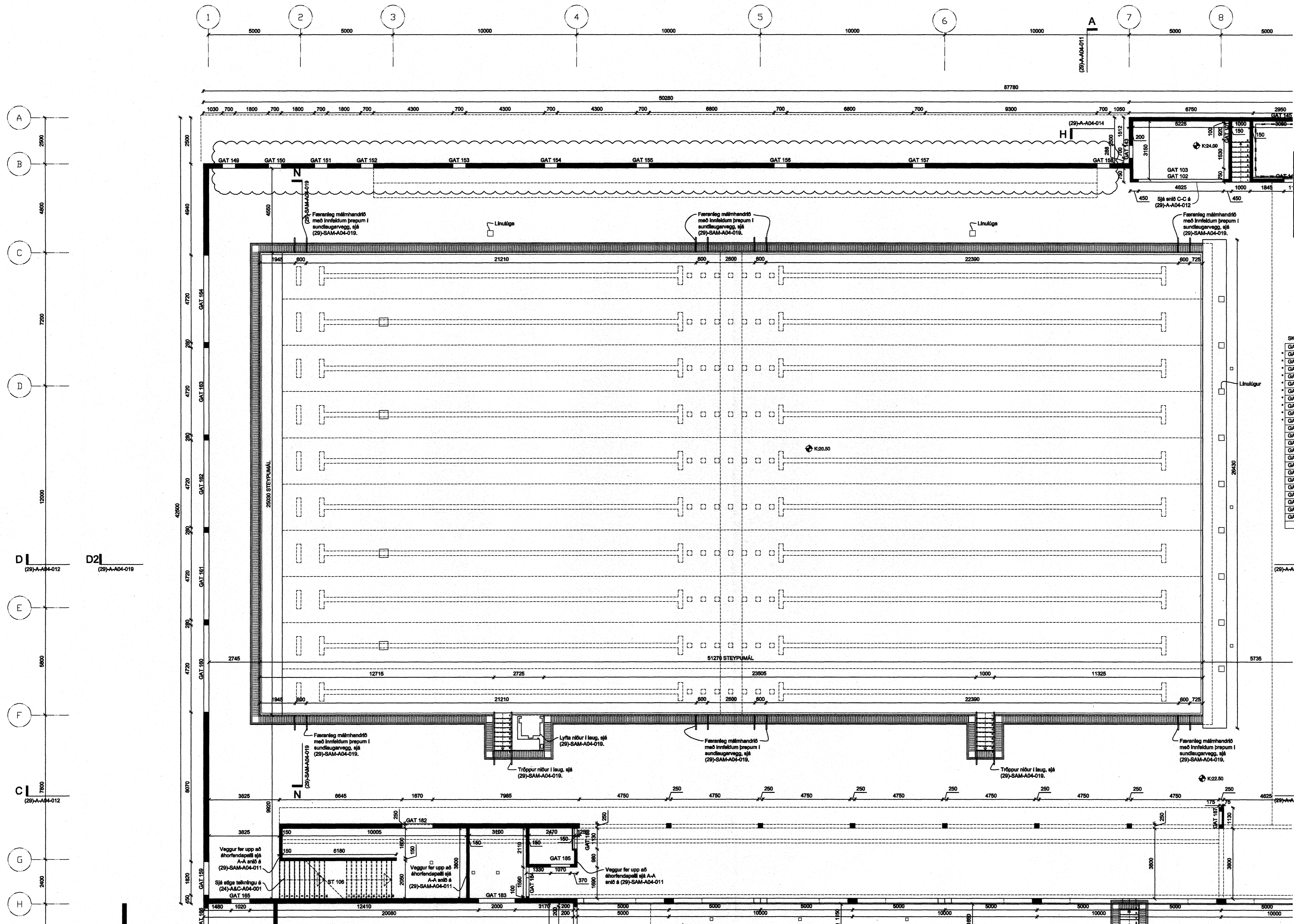
GRUNNMYND 1. HÆÐ MKV.: 1:100
