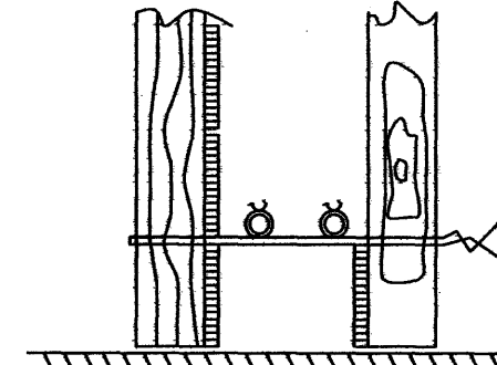
Snið A - A í sökkulvegg Sýnd eru 2 neðstu steypu- styrktarjárn í steypumóti ofan á neðstu mótavírum
