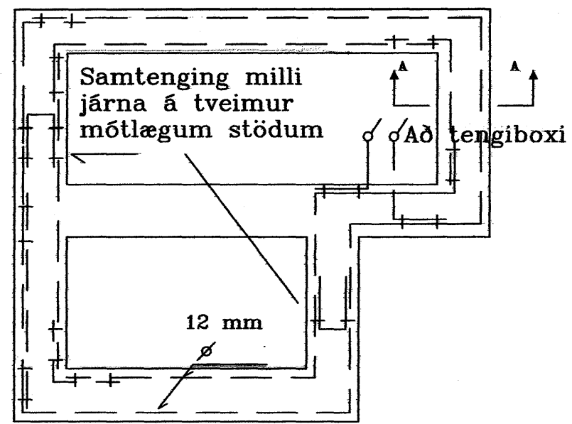
Grunnmynd Sökkulsveggja
