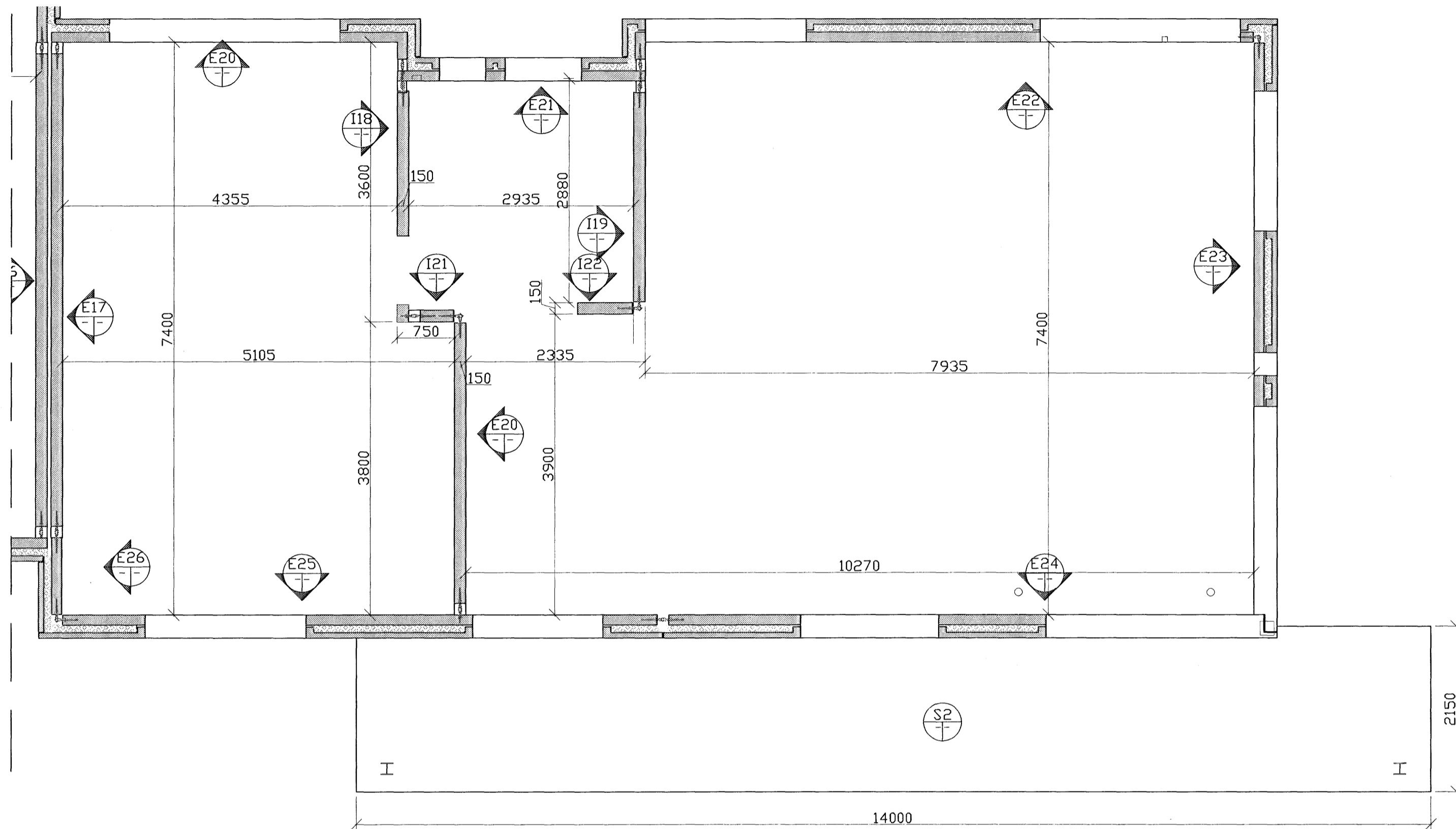
Grunnmynd, 2 hæð Hlíðarás 23 1:50
