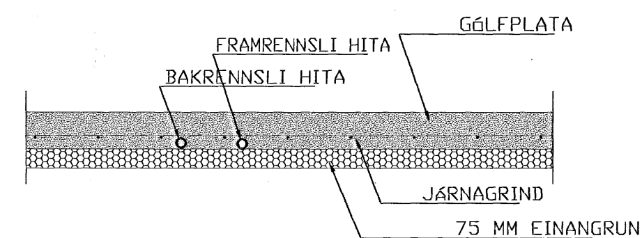
SNID Í HITALAGNIR Í GÖLFI 1:20 RÖR Í RÖR
