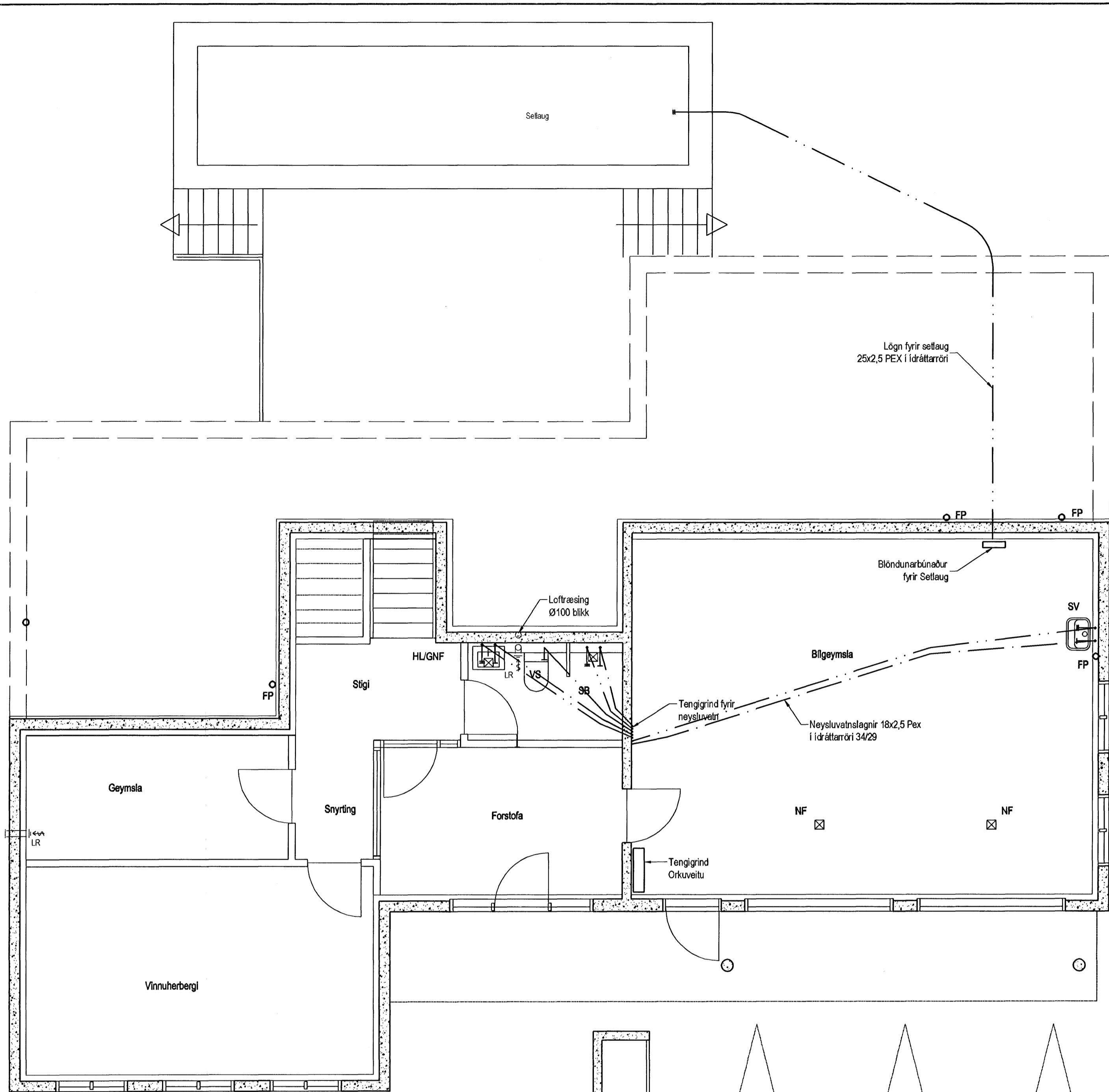
Neysluvatnslagnir 1. hæð, 1:50
