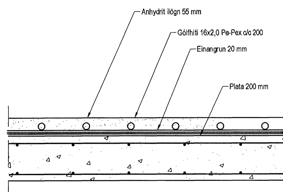
Hita- og vatnslagnir, Snið í milliþötu, 1:10
