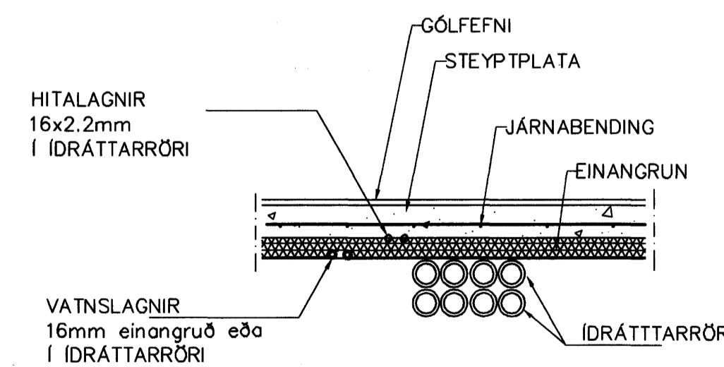
LAGNIR, SNIÐ, 1:20
