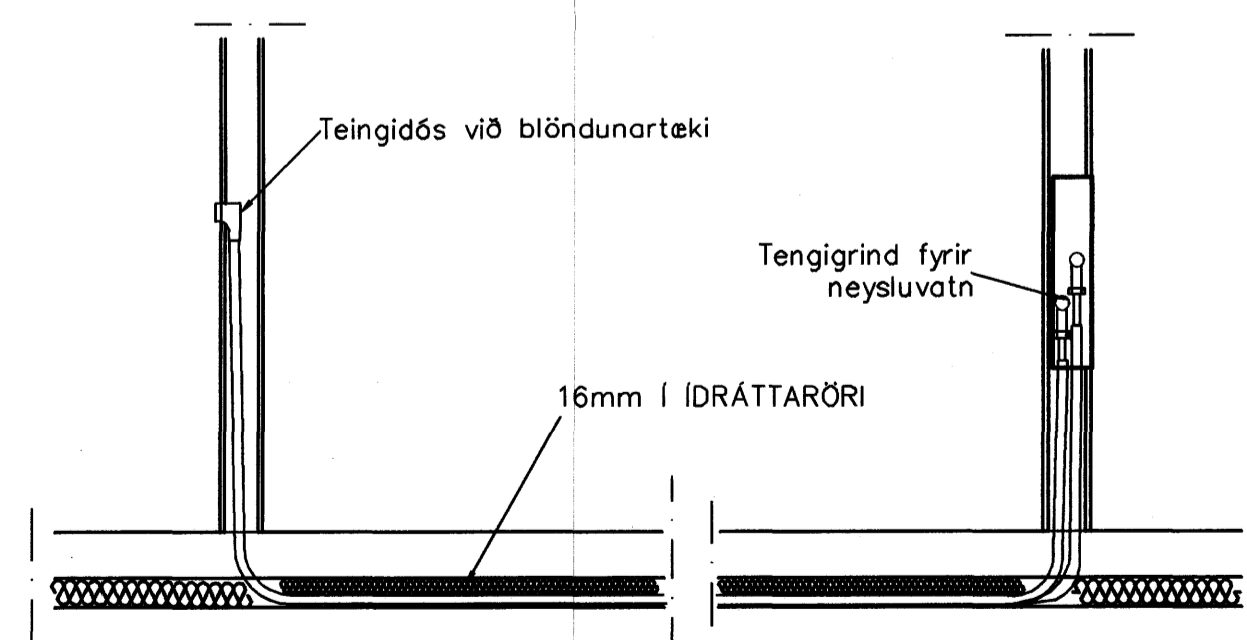
TENGING NEYSLUVATNSLAGNA 1:20
