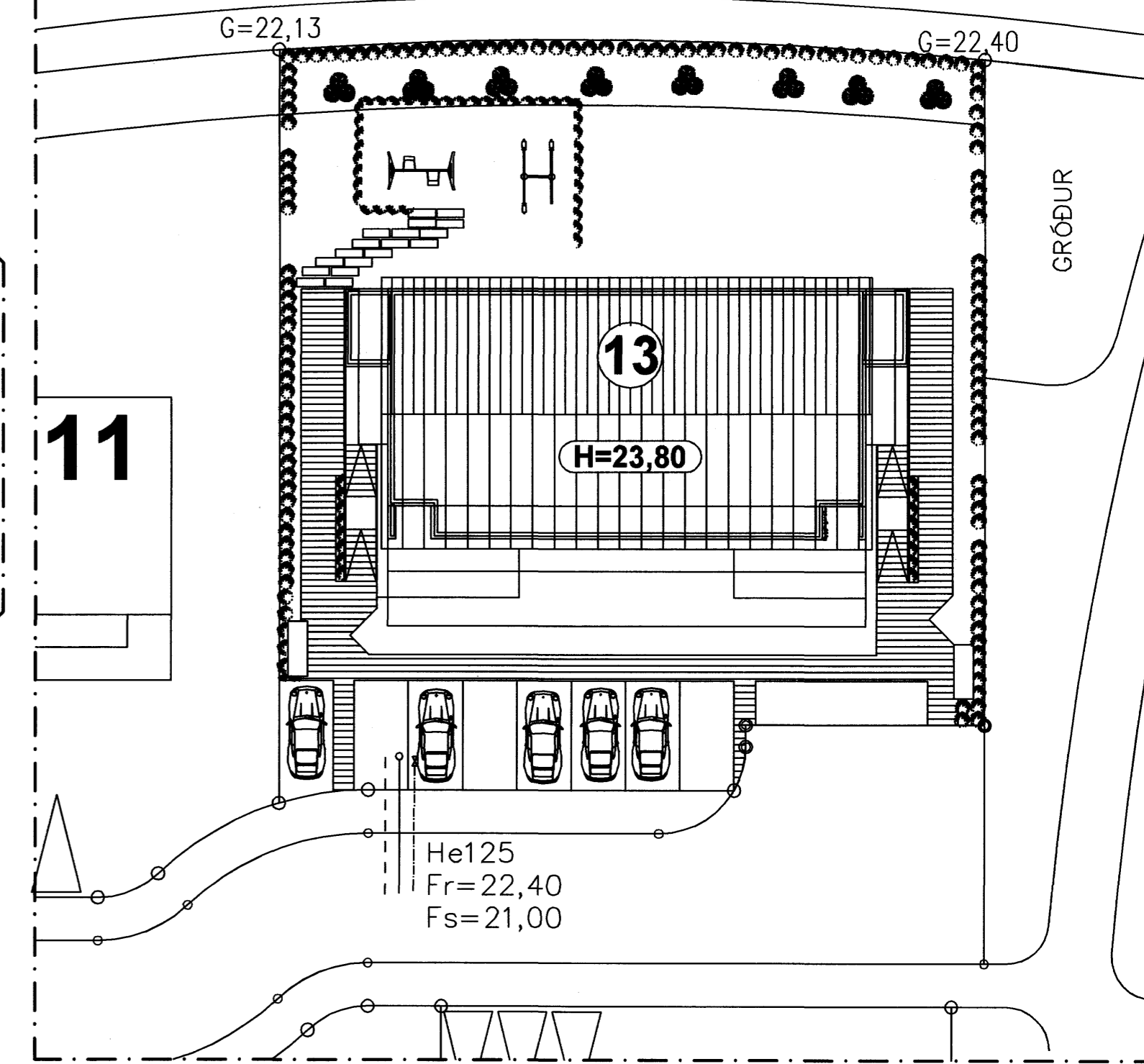
AFSTÖÐUMYND 1:50
