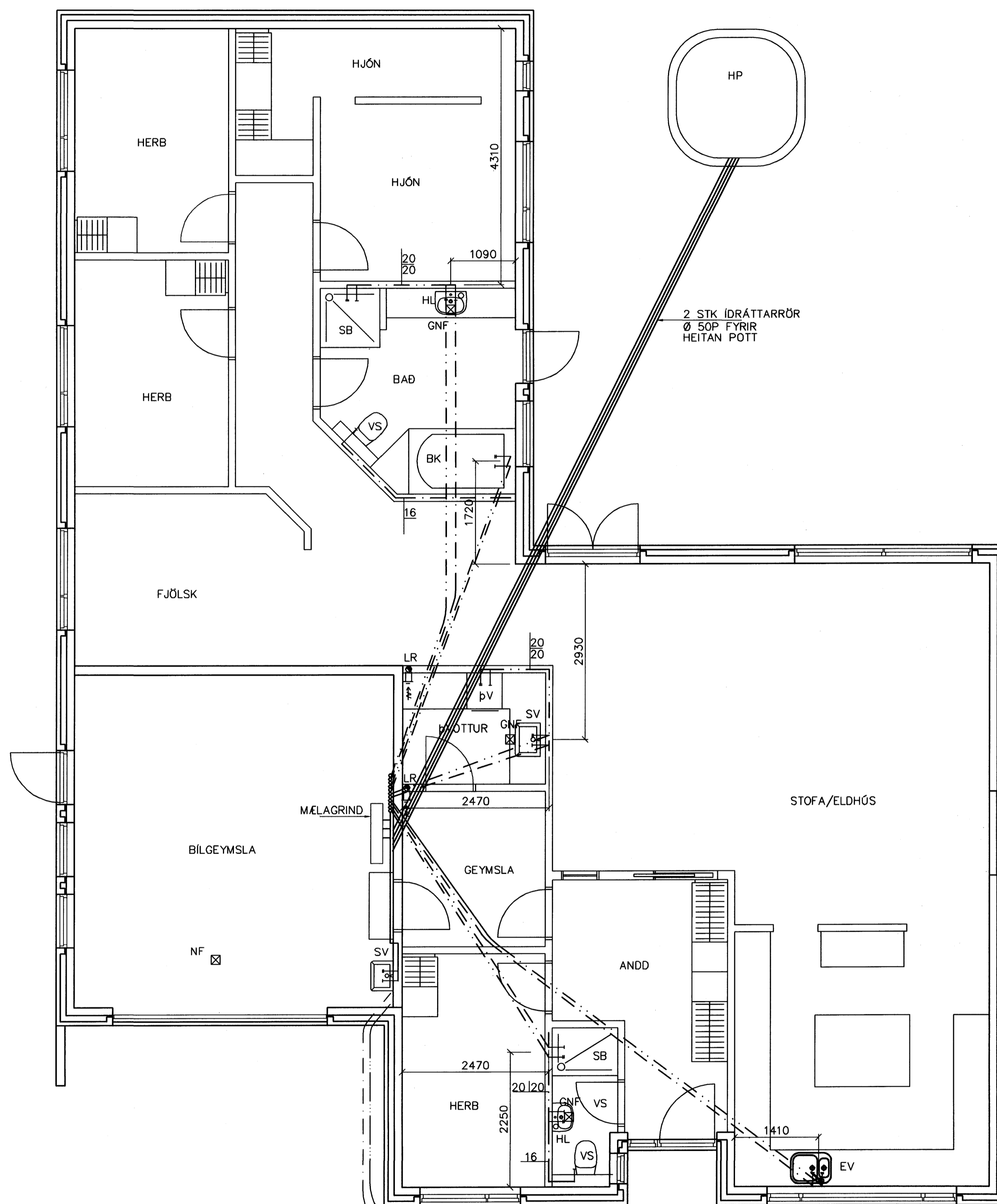
GRUNNMYND 1:50
