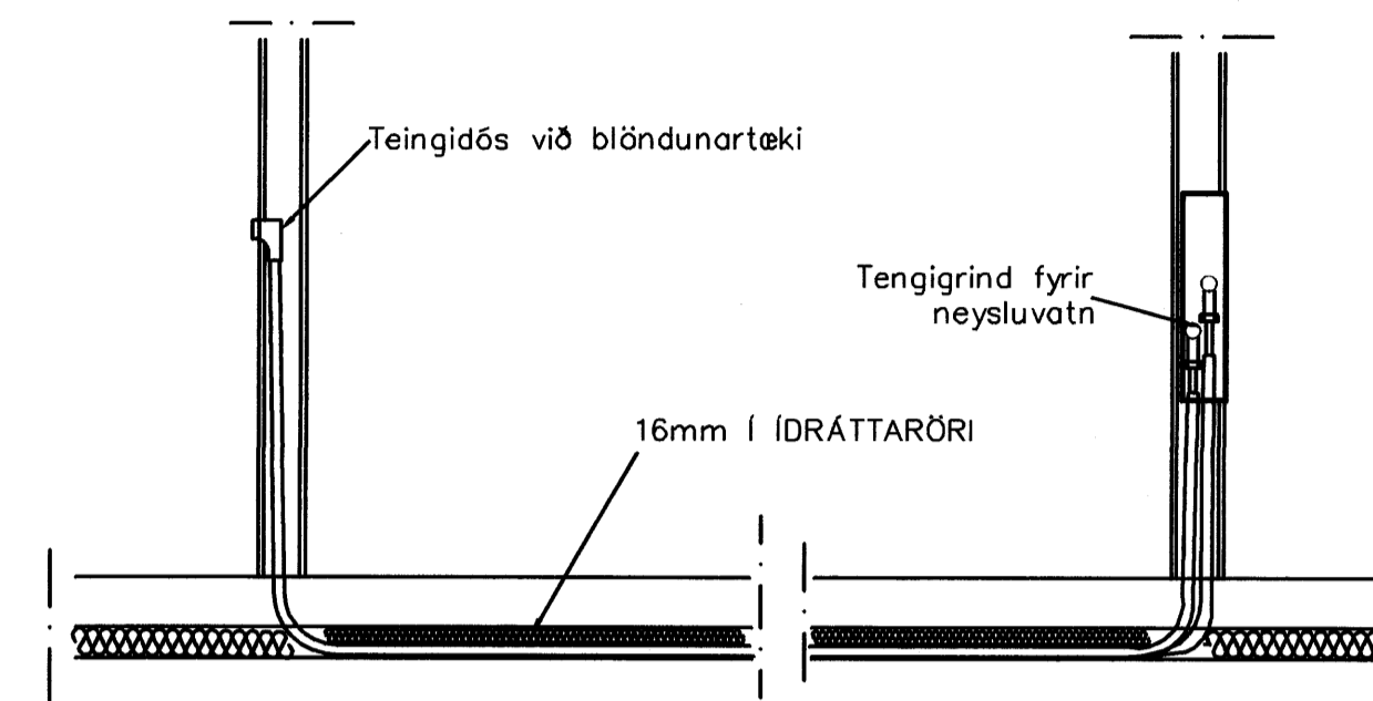
TENGING NEYSLUVATNSLAGNA 1:20
