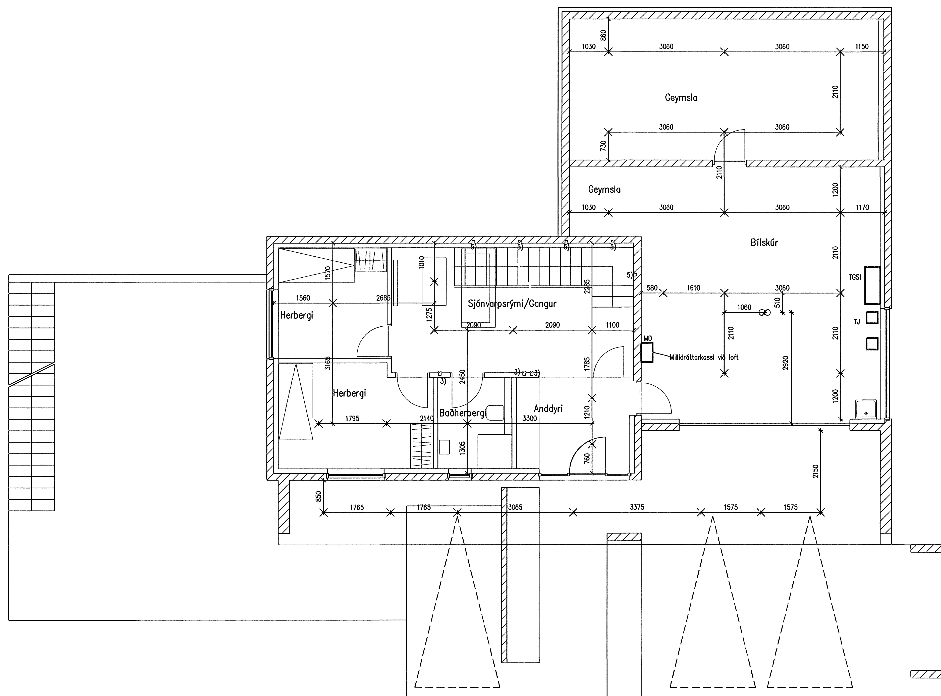
Grunnmynd 1. hæð, 1:50
