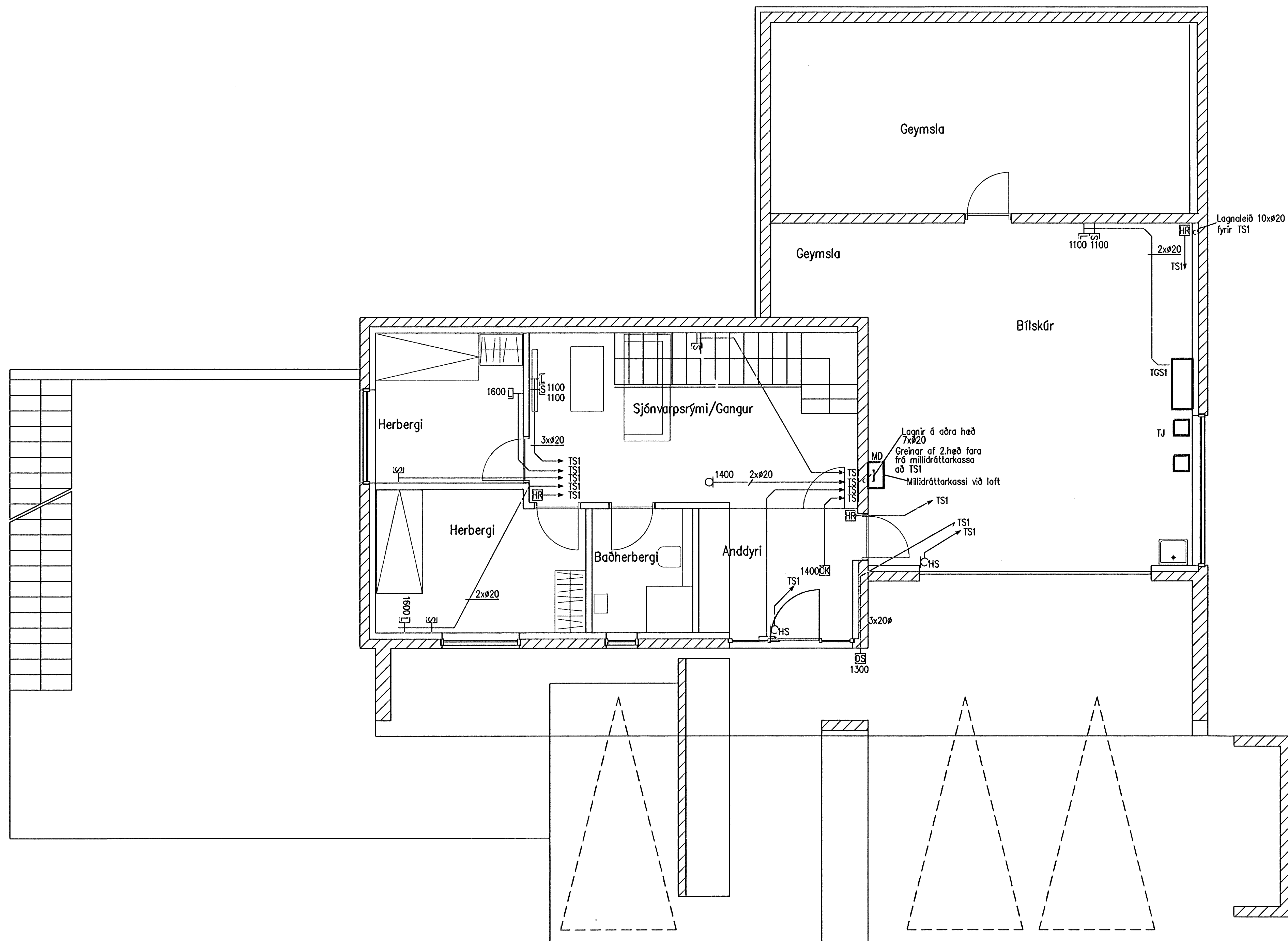
Grunnmynd 1. hæð, 1:50
