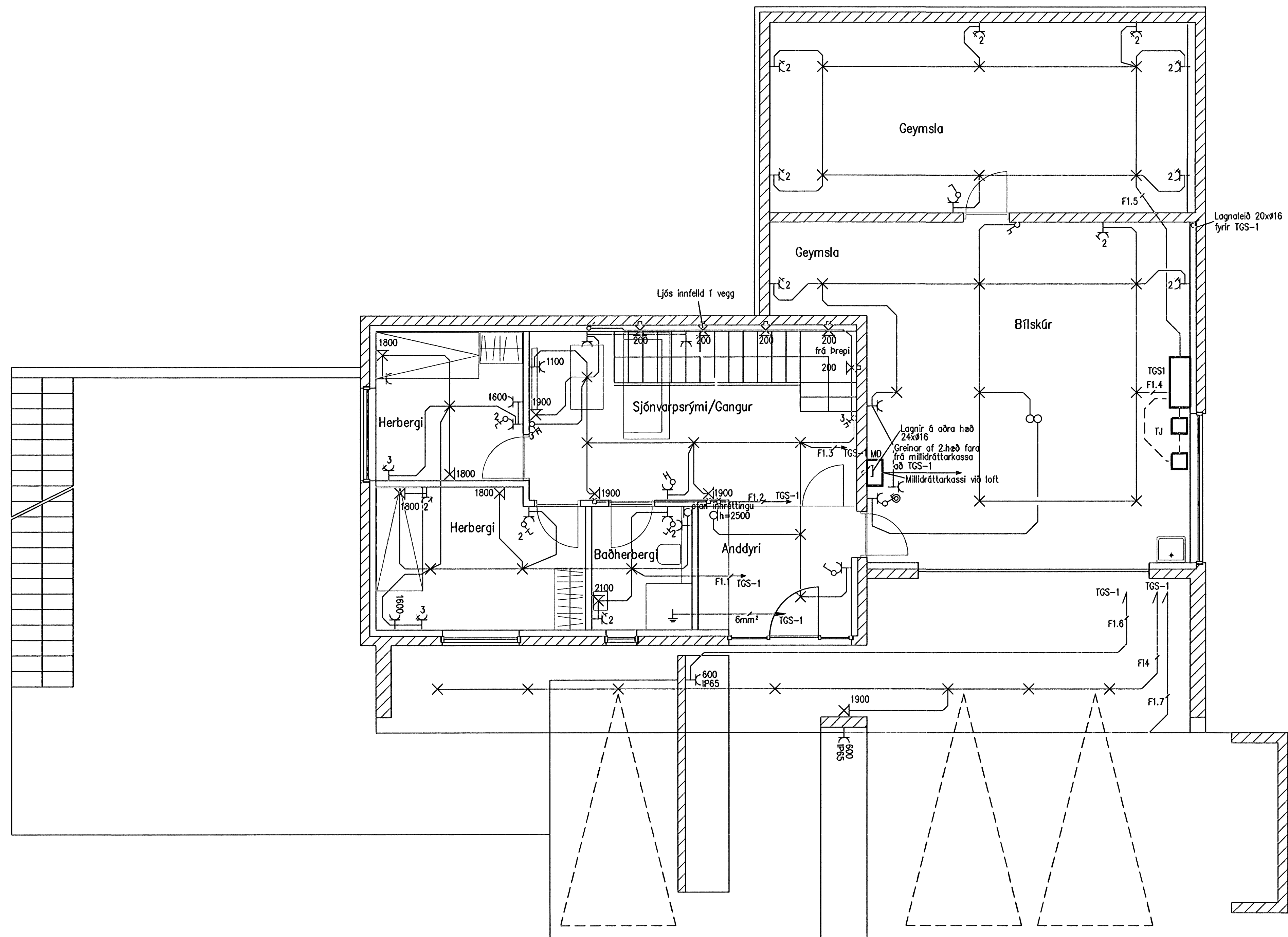
Grunnmynd 1. hæð, 1:50
