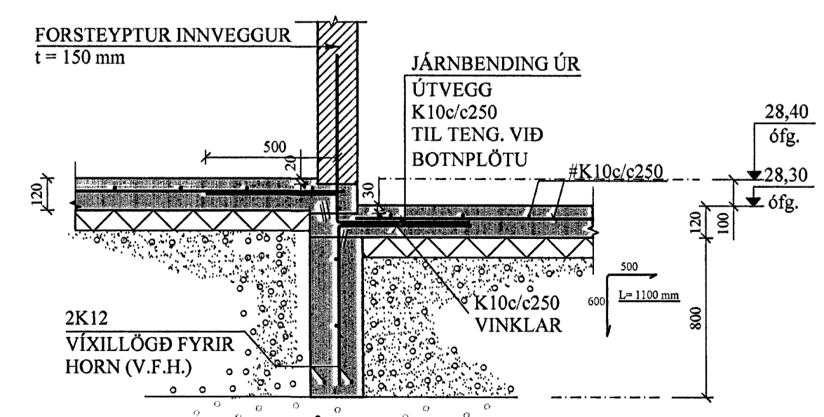
D2 SNÍÐ. 1:20
