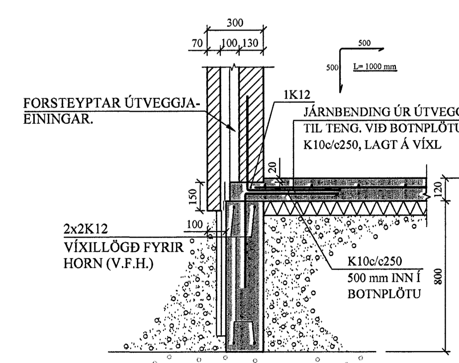
A2 SNÍÐ. 1:20
