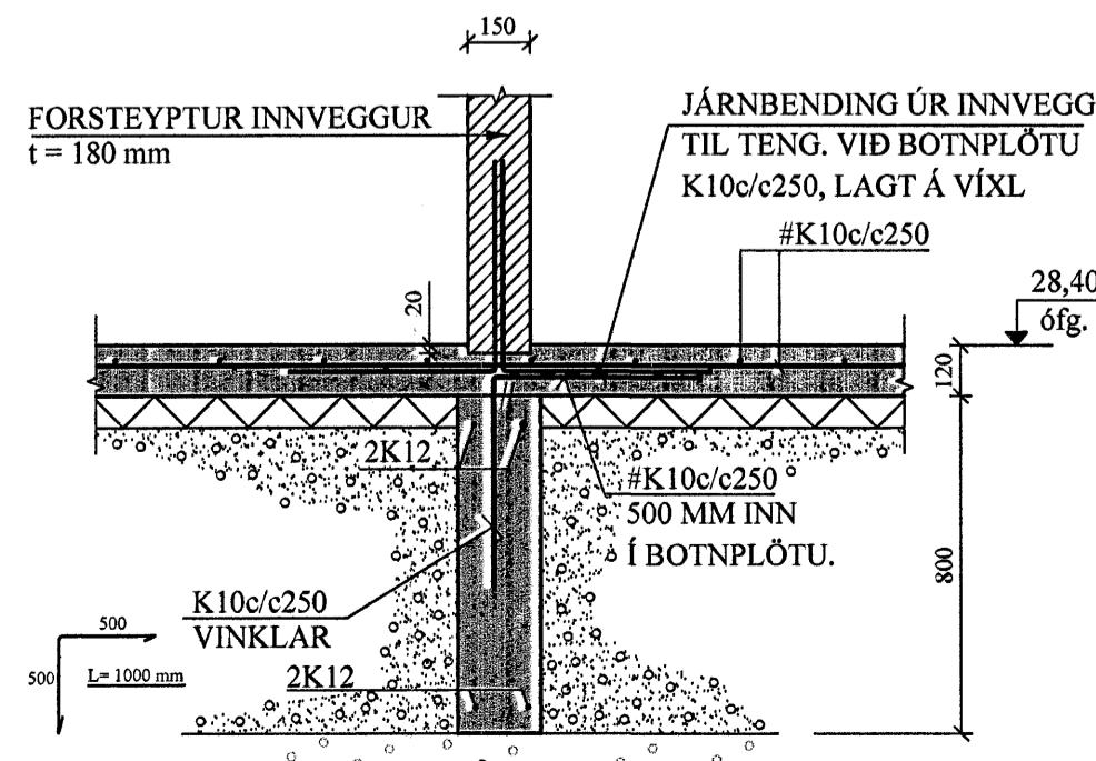
C2 SNÍÐ. 1:20
