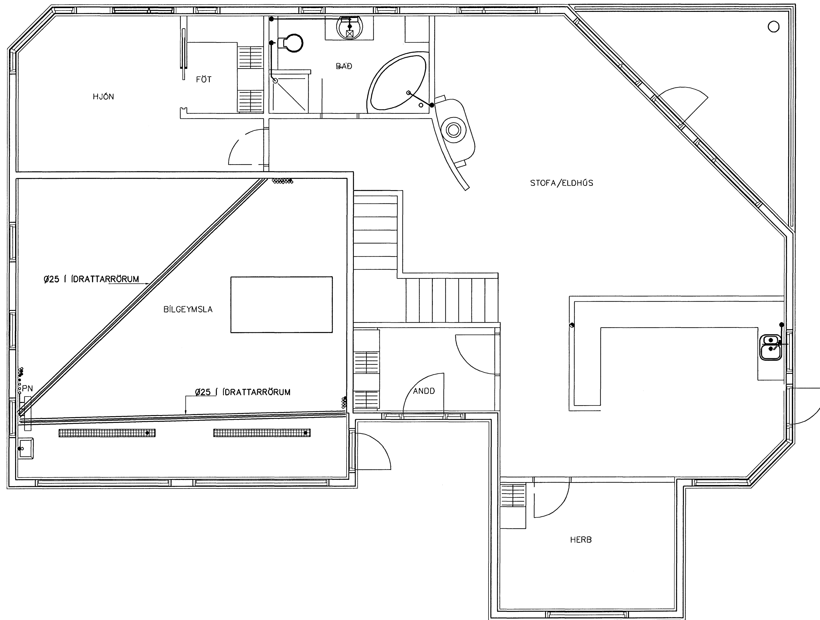
GRUNNMYND 2. HÆÐAR 1:50
