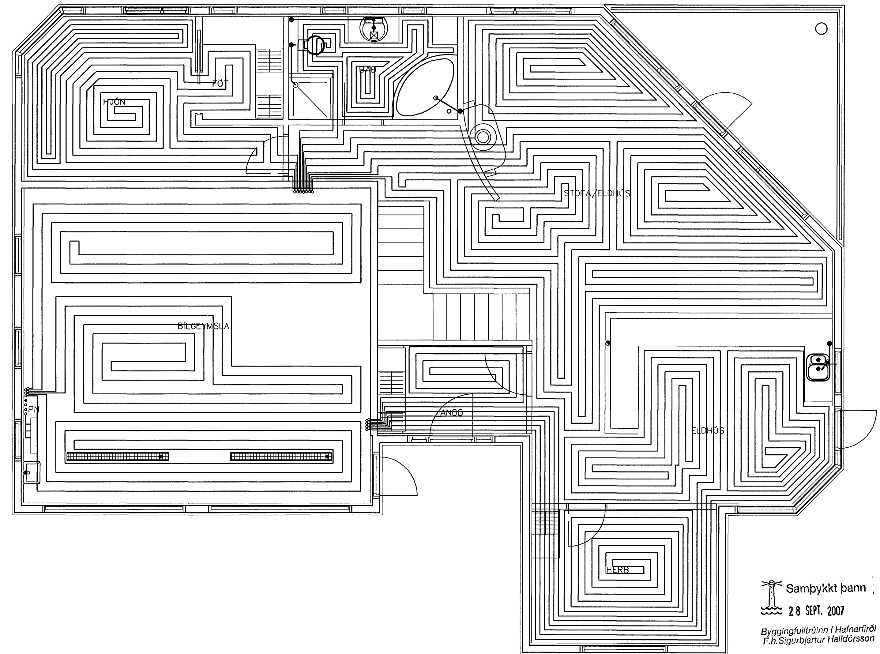
GRUNNMYND 2. HÆÐAR 1:50
