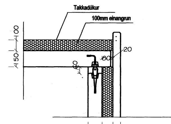
Snið E10 1:20
