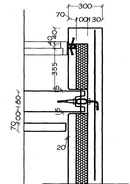
Snið E12 1:20
