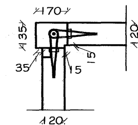
Snið E11 1:20
