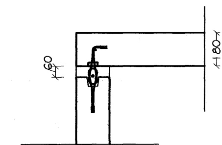
Snið E5 1:20
