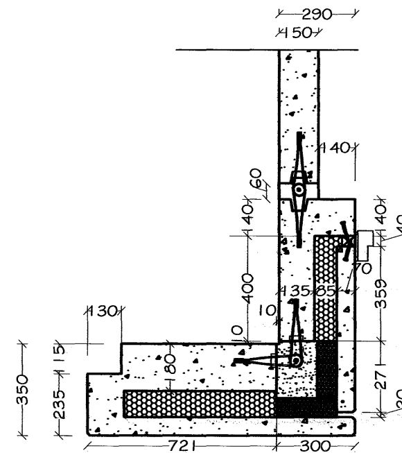
Snið E3 1:20
