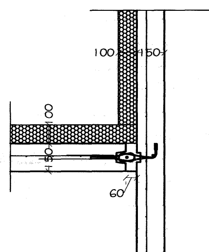
Snið E7 1:20
