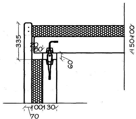
Snið E6 1:20
