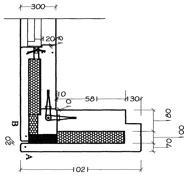
Snið E2 1:20
