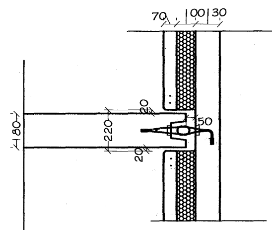
Snið E4 1:20
