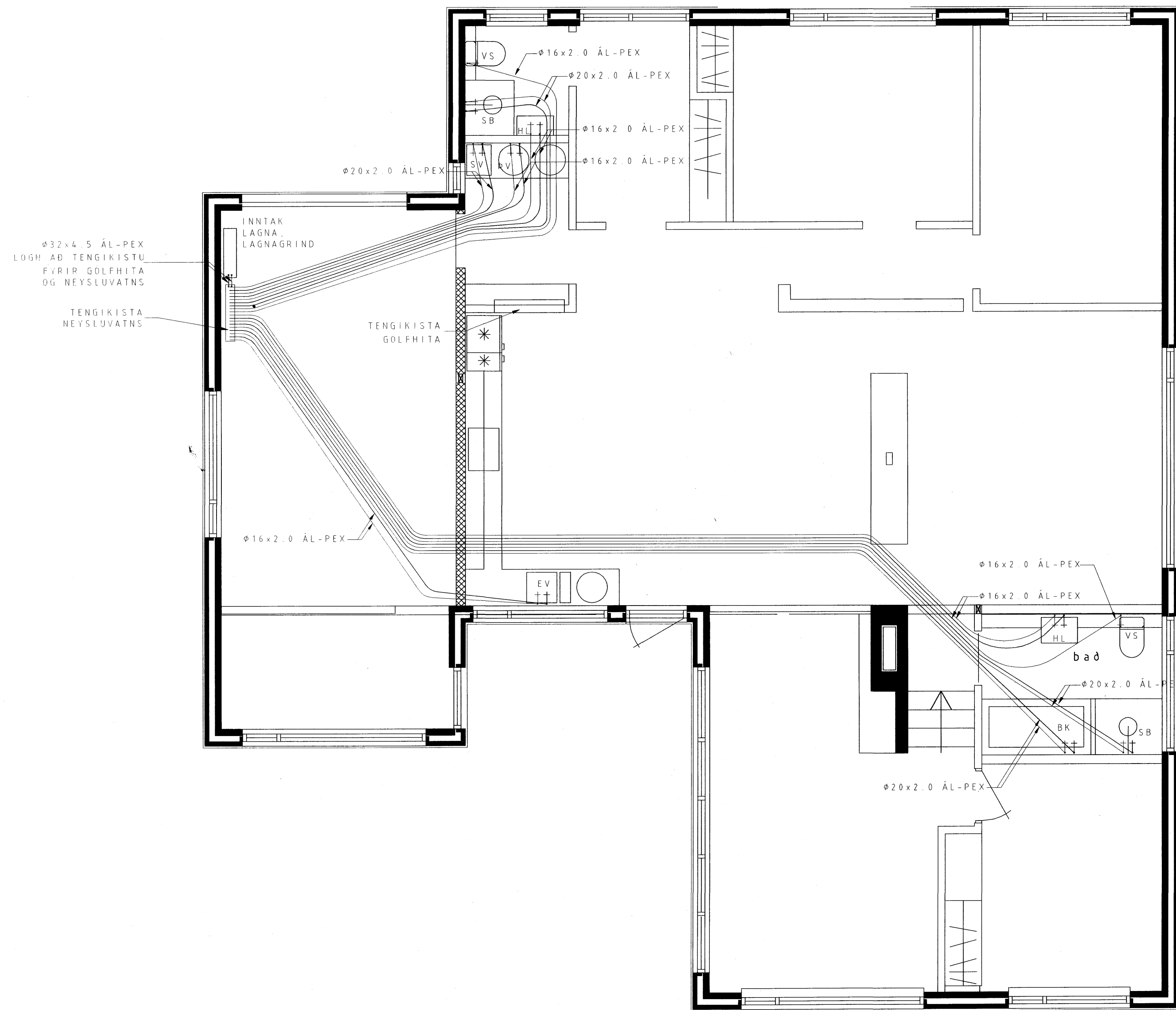
GRUNNMYND NEYSLUVATNS 1:50
