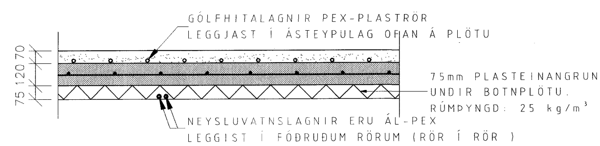
SNIÐ LAGNIR Í BOTNPLÖTU 1:20
