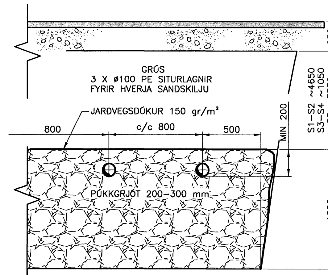
SNID Í DRENLAGNIR/SITURLAGNIR 1:20
