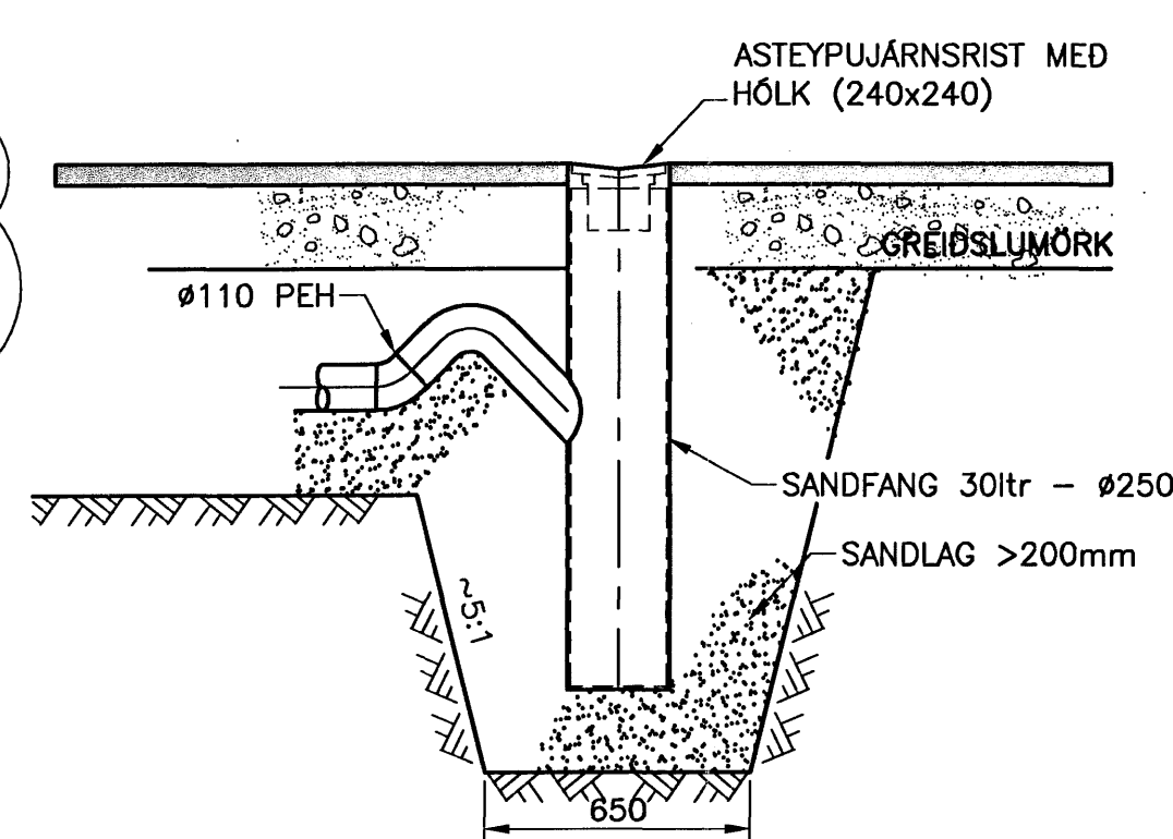
NIDURFÖLL – Ø250 1:20
