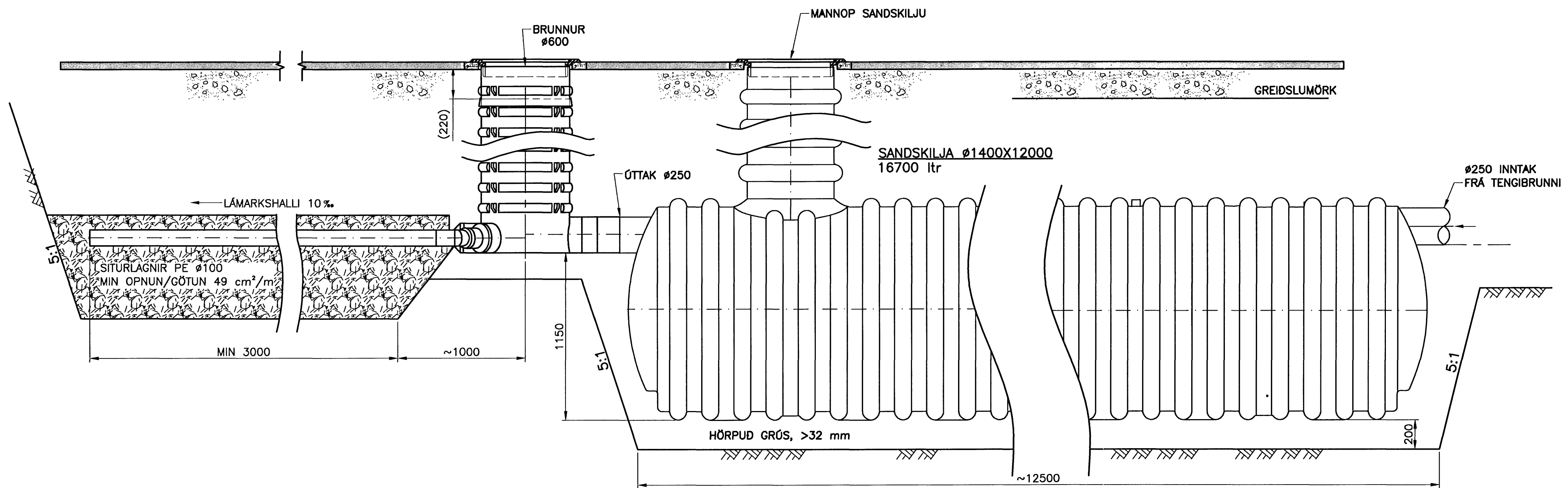
SANDSKILJA OG DRENLAGNIR – LANGSNID 1:20
