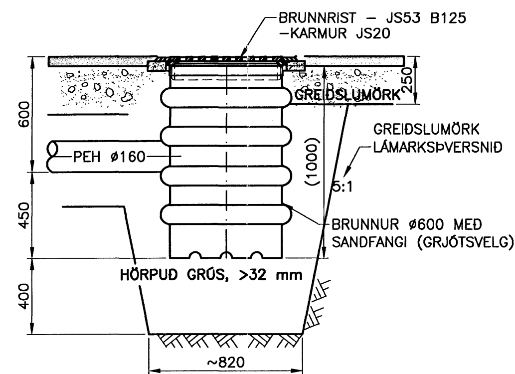
NIDURFÖLL – Ø600 1:20
