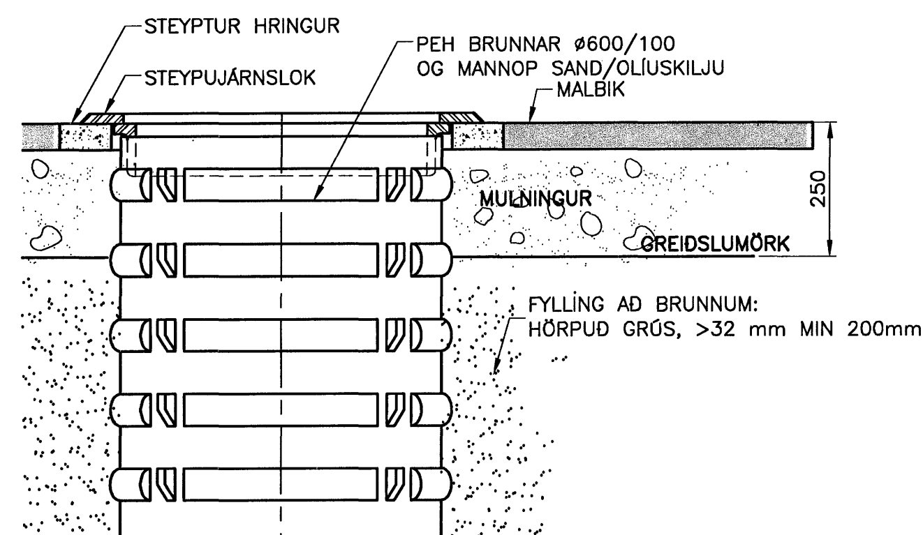
FRÁGANGUR BRUNNA 1:10
