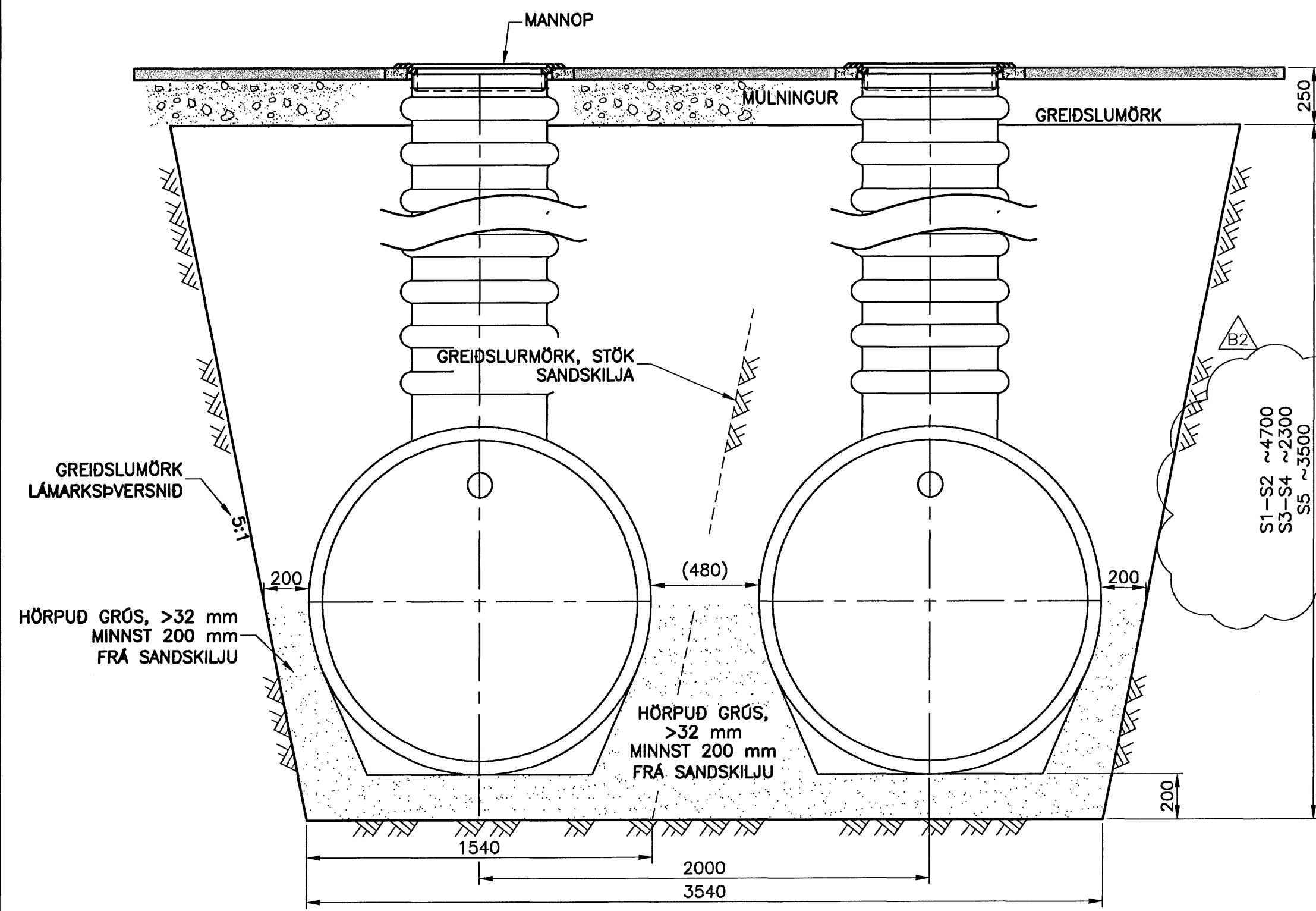
ÞVERSNID Í SANDSKILJUR 1:20
