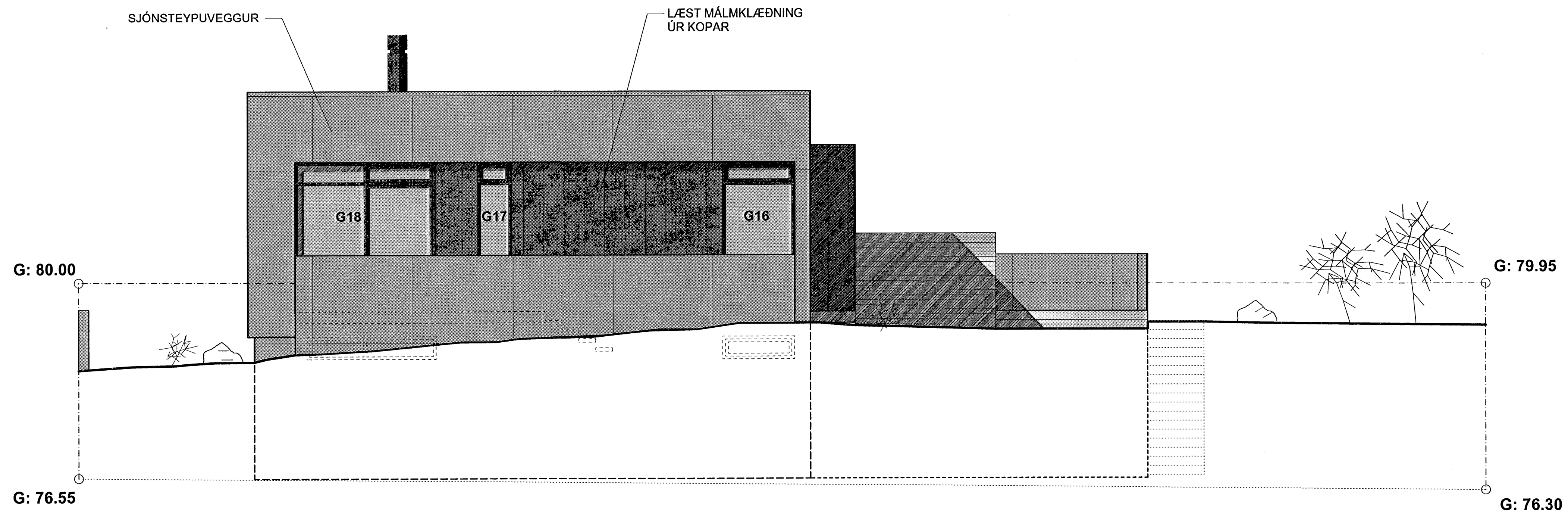
ÚTLIT VESTUR -með steypu handriði/vegg
