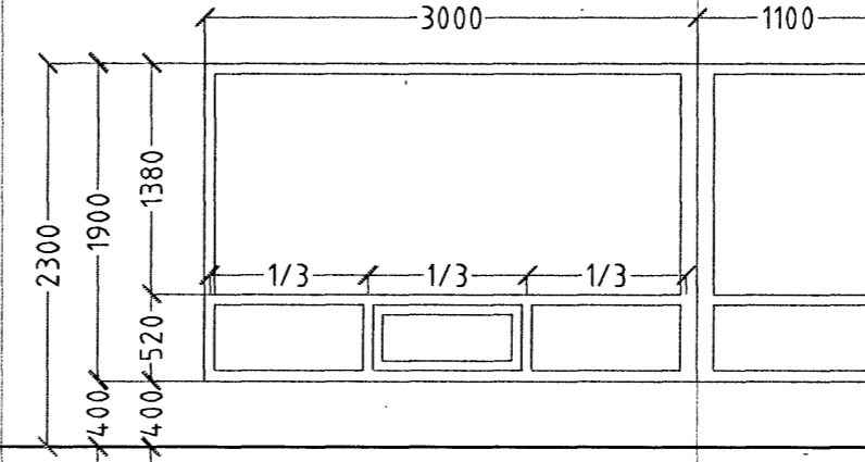
1 STK. Stofa. Horngluggi
