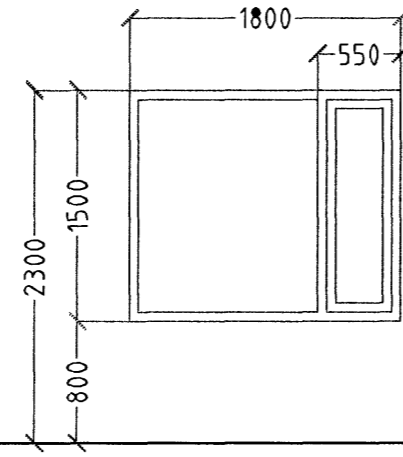
3 STK. Herb. Björgunarop
