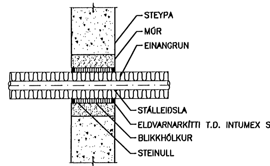
BRUNARÞÉTTING Á LEIDSLU GEGNUM STEYPTAN VEGG EKKI Í KVARÐA
