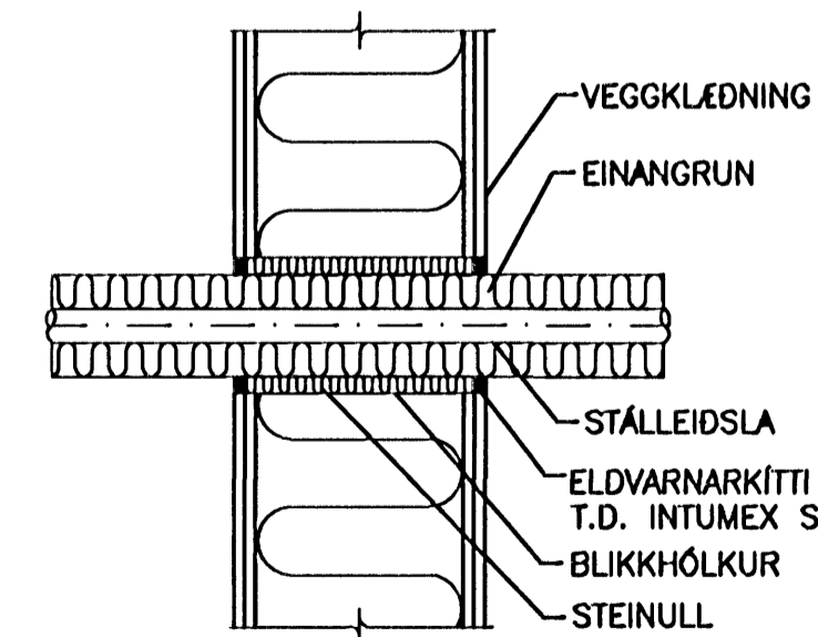
BRUNARÞÉTTING Á LEIDSLU GEGNUM LÉTTAN VEGG EKKI Í KVARÐA
