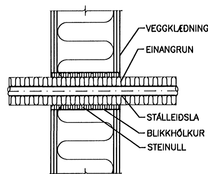
ÞÉTTING Á STÁL-/PEXLEIDSLU GEGNUM LÉTTAN VEGG EKKI Í KVARÐA
