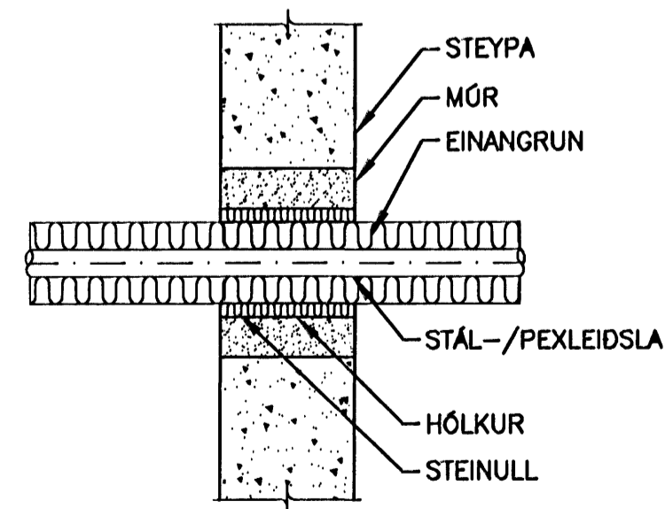
ÞÉTTING Á STÁL-/PEXLEIDSLU GEGNUM STEYPTAN VEGG MKV.2
