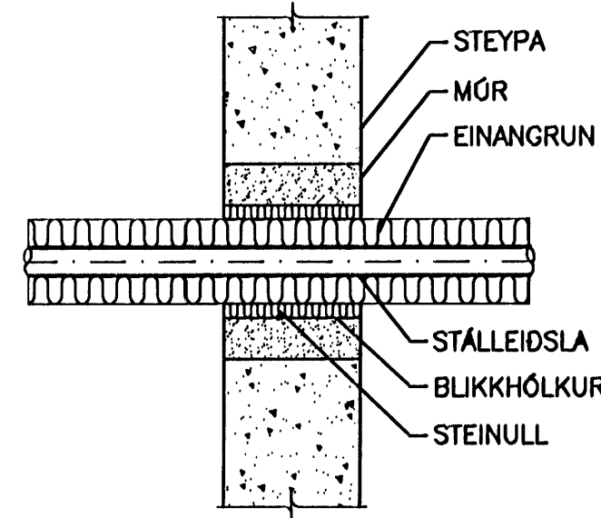
ÞÉTTING Á STÁL-/PEXLEIÐSLU GEGNUM STEYPTAN VEGG
