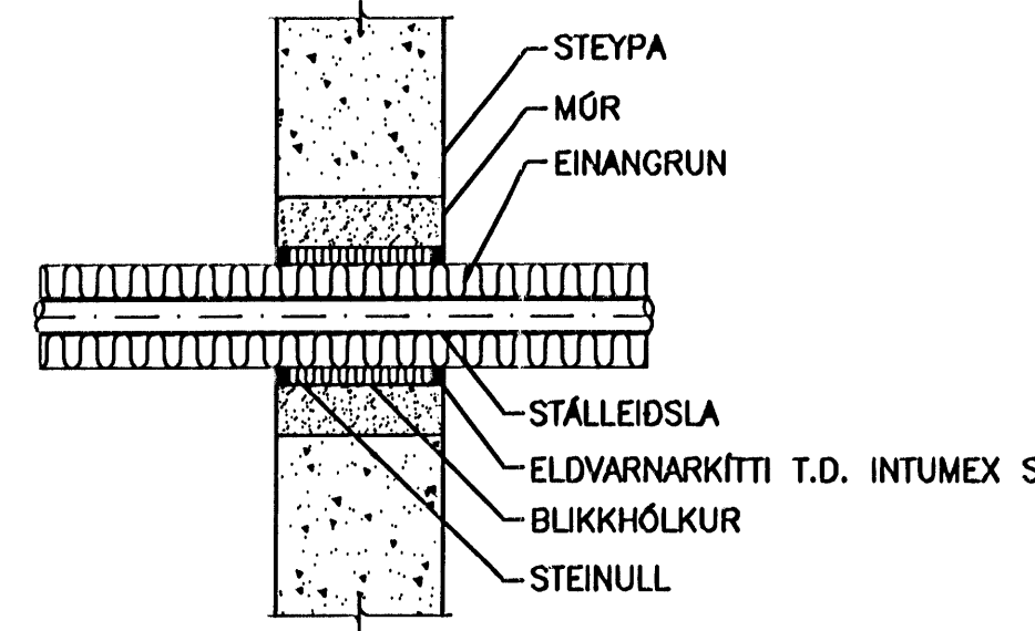
BRUNAPÉTTING Á LEIÐSLU GEGNUM STEYPTAN VEGG
