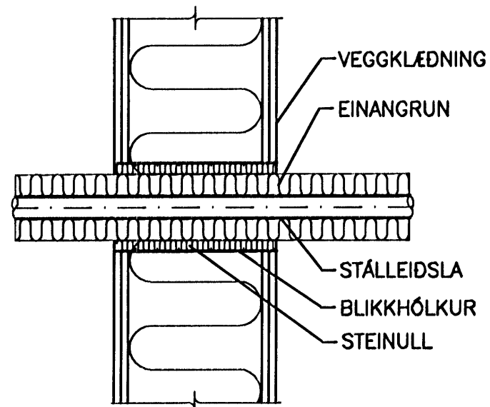
ÞÉTTING Á STÁL-/PEXLEIÐSLU GEGNUM LÉTAN VEGG
