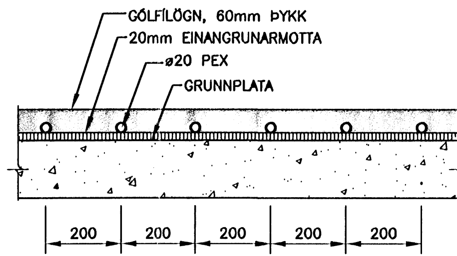
SNID I GÖLFHITALÖGN MKV. 1
