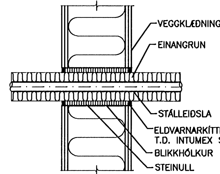
BRUNAPÉTTING Á LEIÐSLU GEGNUM LÉTAN VEGG MKV. 1
