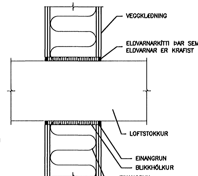
FRÁGANGUR Á LOFTSTOKKUM GEGNUM LÉTTAN VEGG EKKI Í KVARDA
