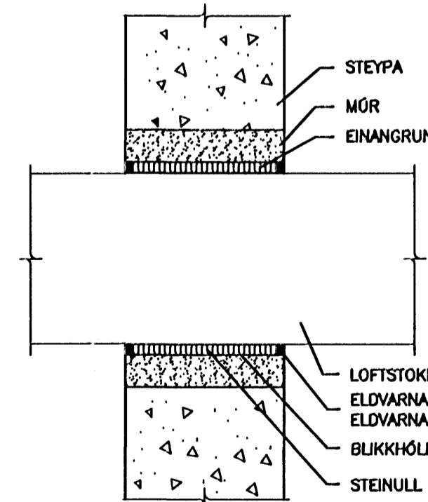
FRÁGANGUR Á LOFTSTOKKUM GEGNUM STEYPTA VEGGI OG PLÖTUR EKKI Í KVARDA
