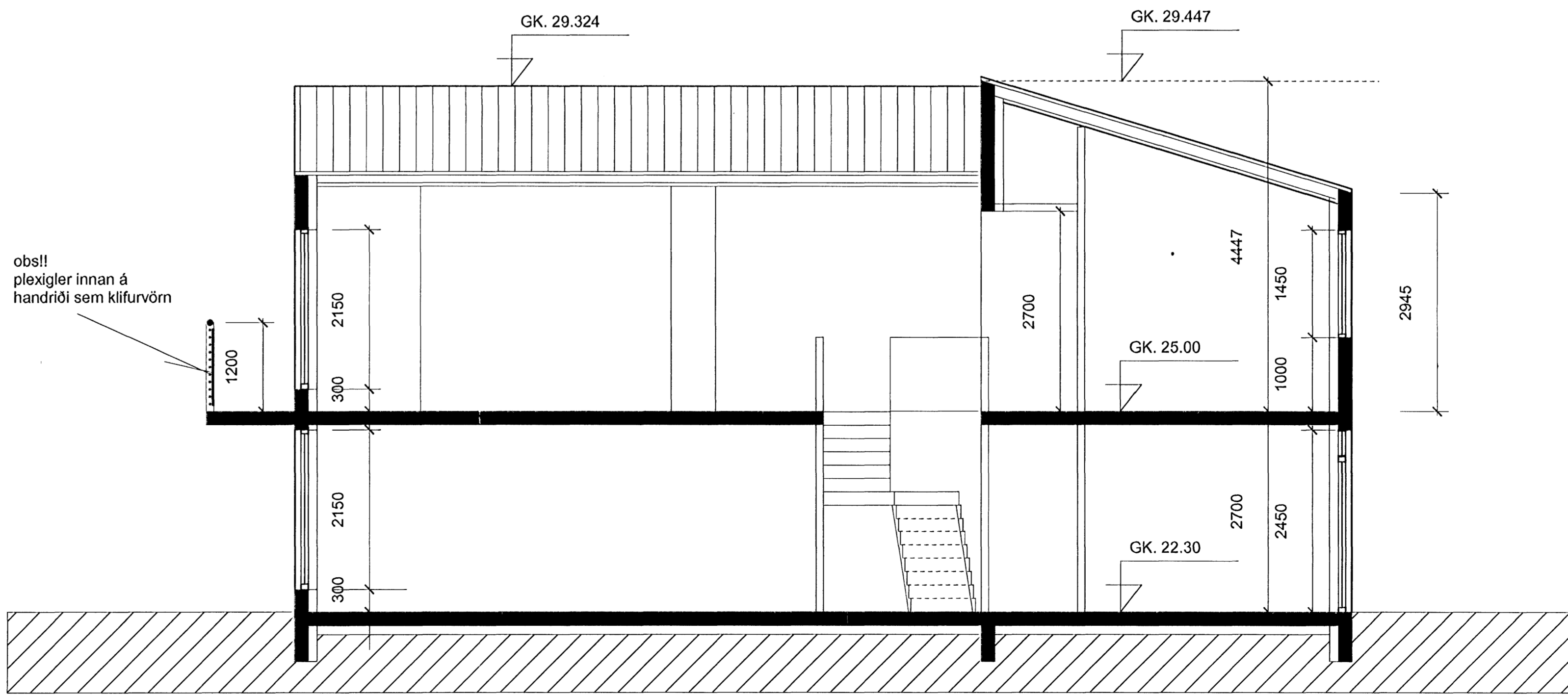
Sneiðing A-A
