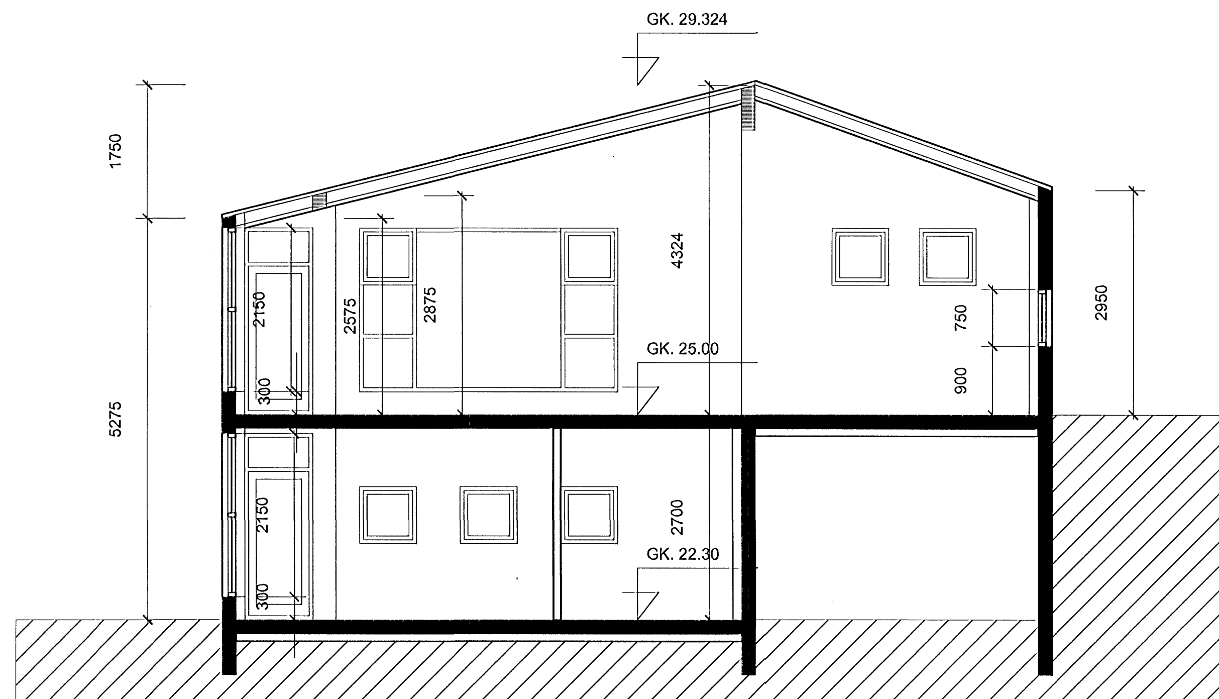
Sneiðing B-B
