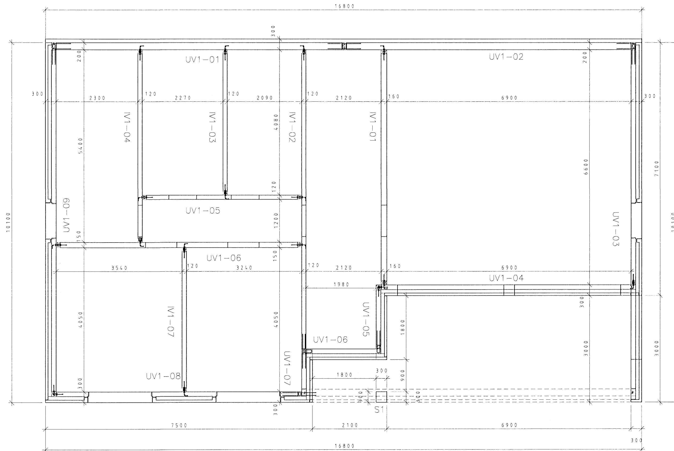
GRUNNMYND 1. HÆÐAR 1:50
