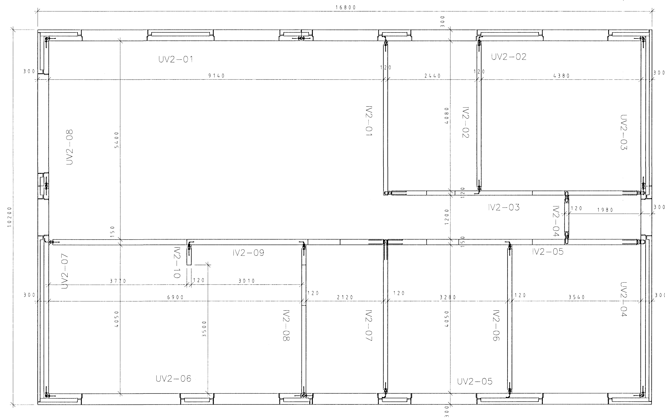
GRUNNMYND 2. HÆÐAR 1:50
