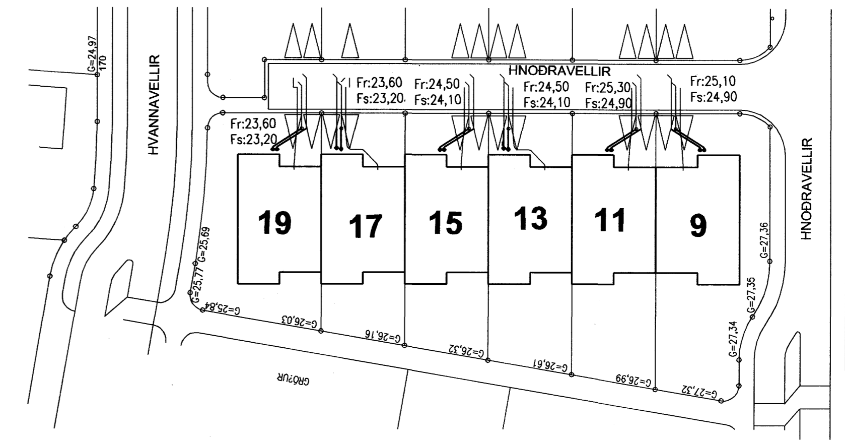
Afstöðumynd, 1:500
