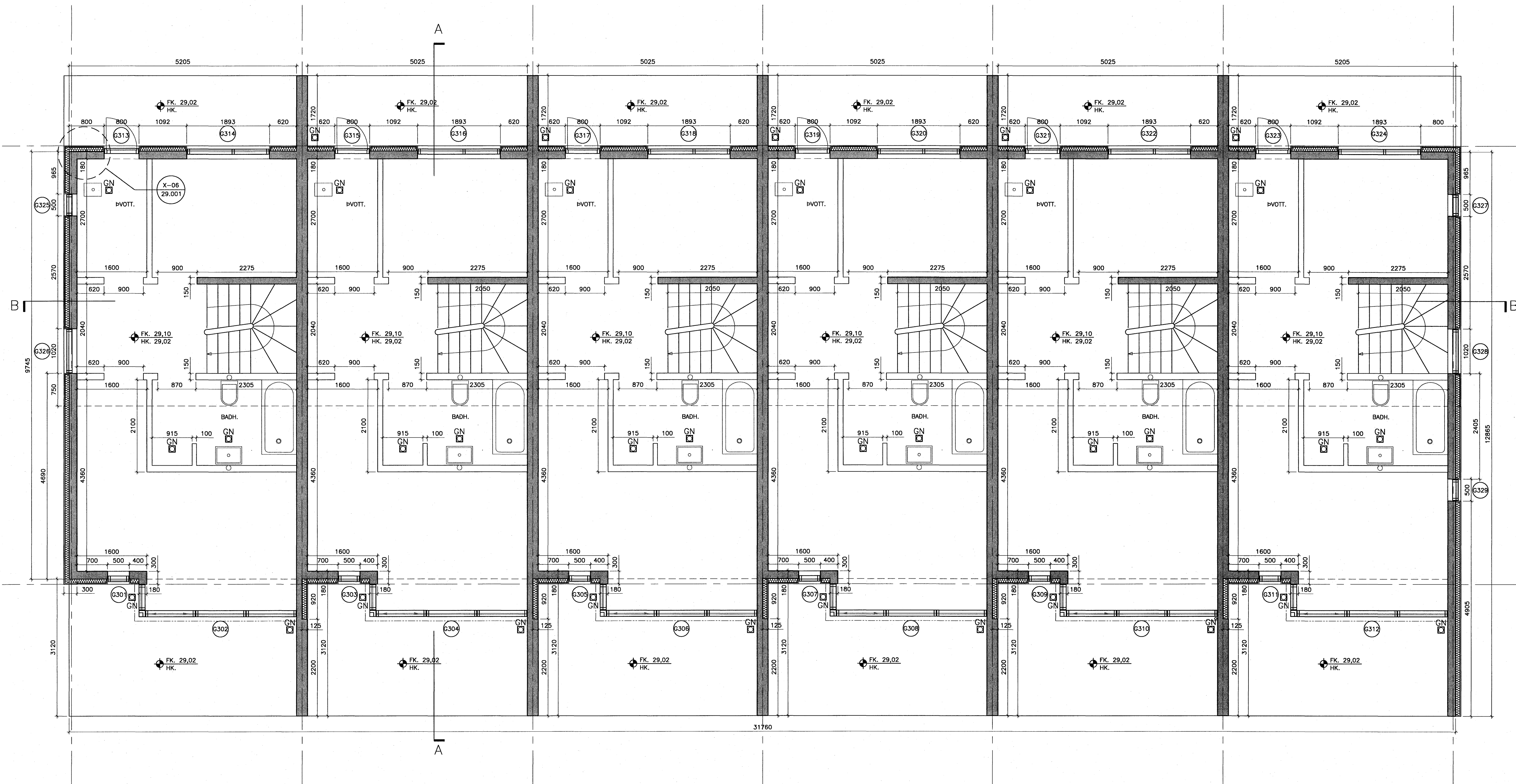
GRUNNMYND 3. HÆÐAR KVARDI 1:50
