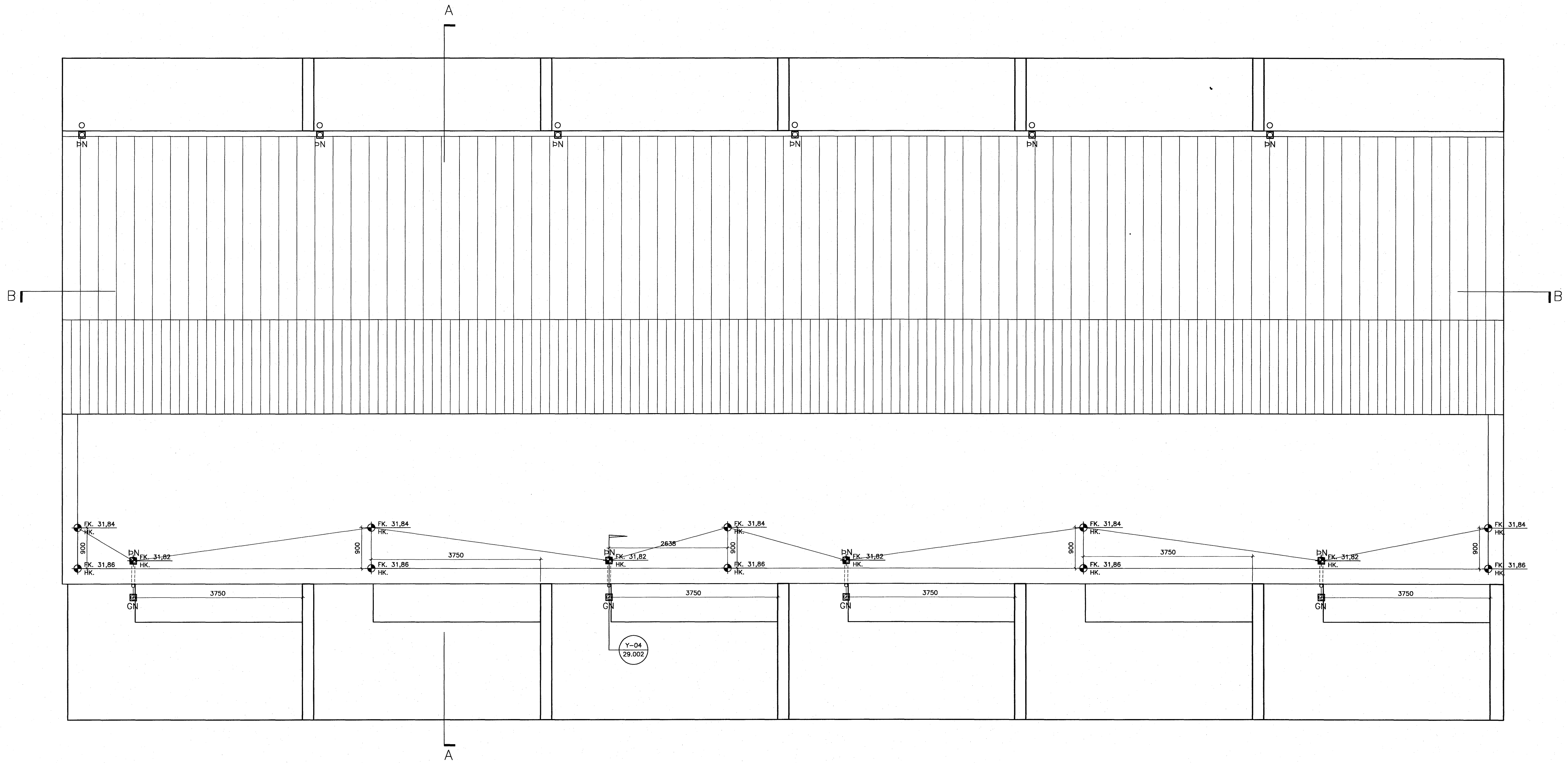
GRUNNMYND ÞAKS KVARDI 1:50
