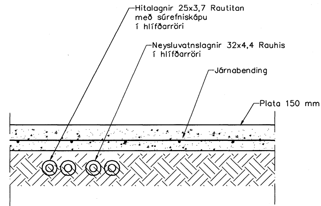
Hita- og Neysluvatnslagnir, Snið í botnplötu, 1:10
