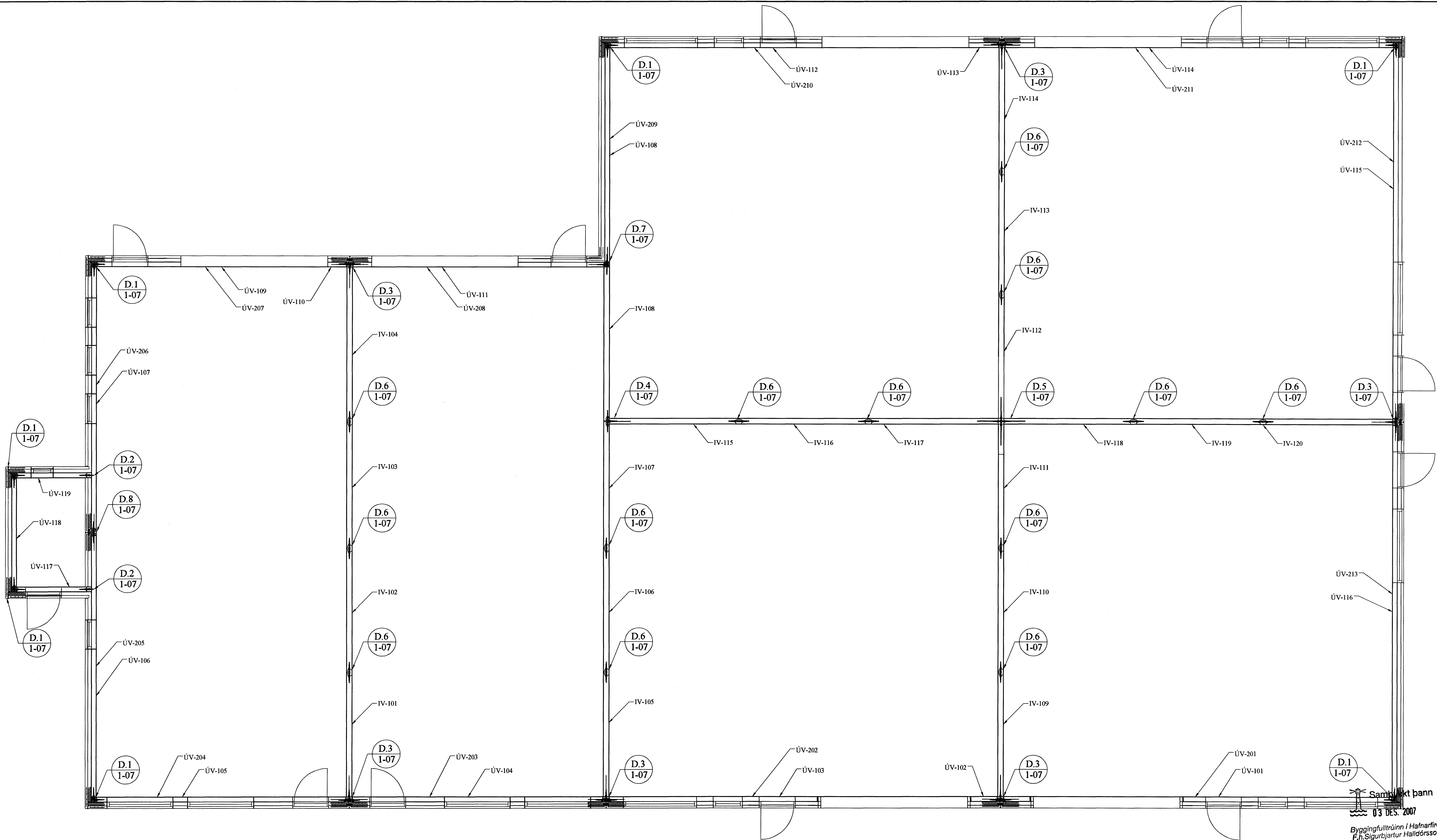
Veggeiningar Grunnmynd, 1:50
