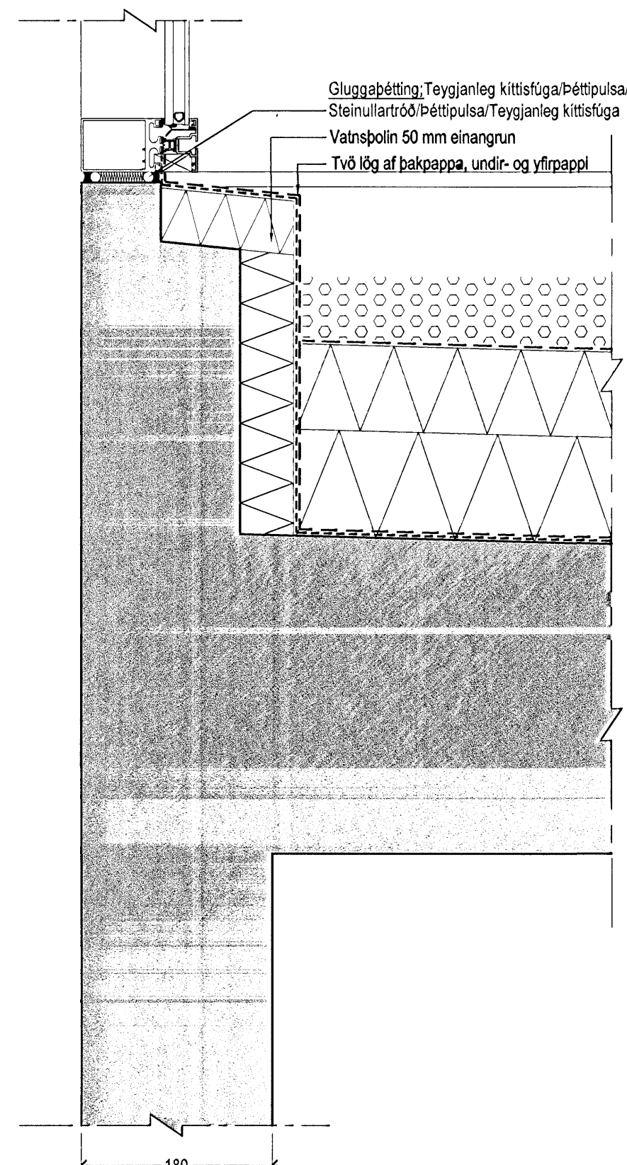
DEILI 1 - Frágangur við þakglugga
