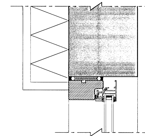
DEILI 3 - Frágangur við yfir- og hliðarstykki glugga
