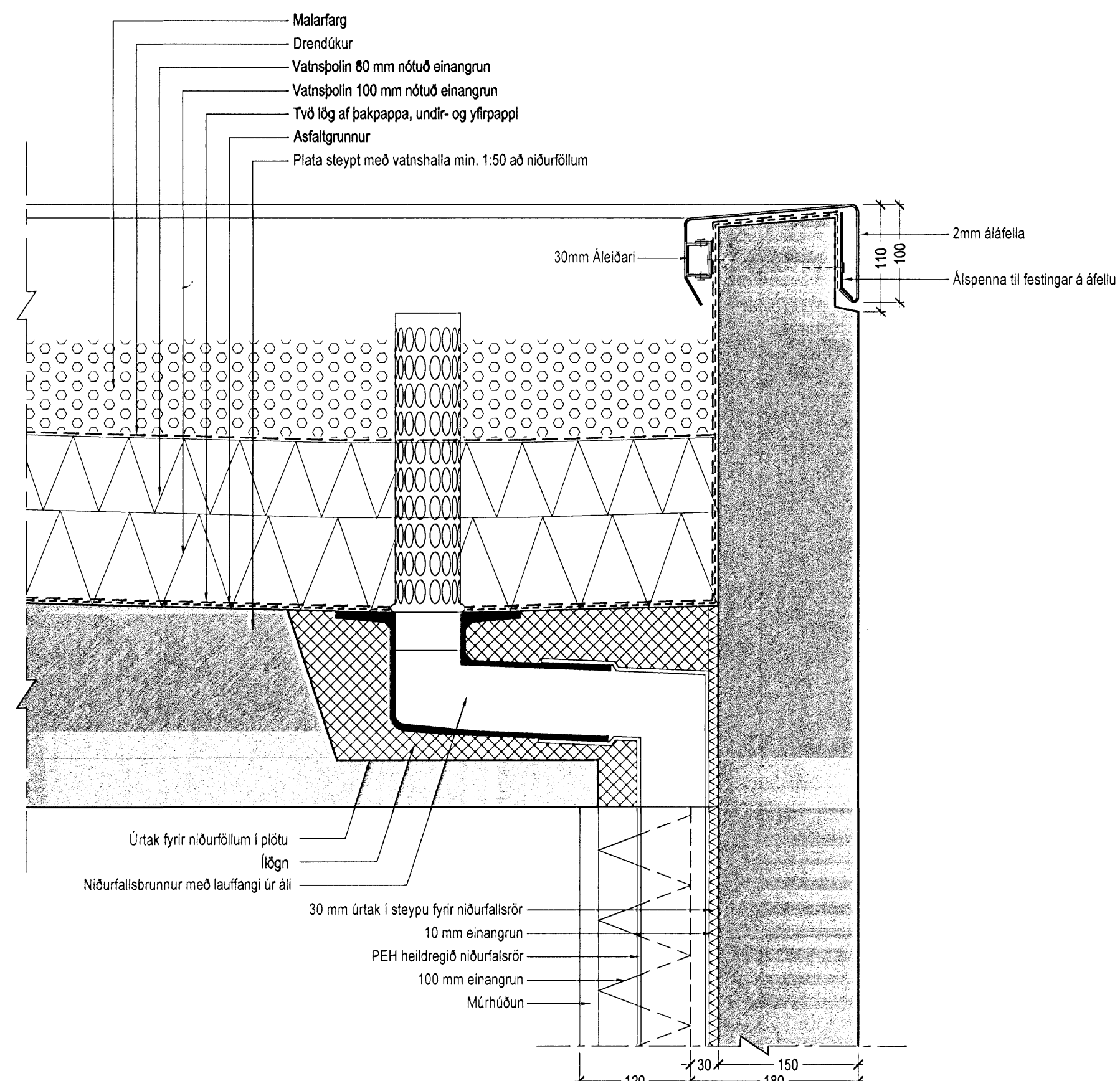
DEILI 2 - Frágangur þaks við útrún og niðurfall
