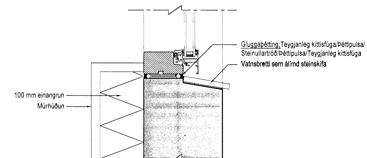
DEILI 4 - Frágangur við botnstykki glugga
