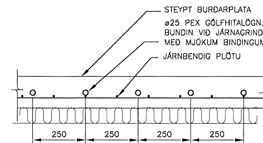
SNID Í GÓLFHITALÖGN 1:10
