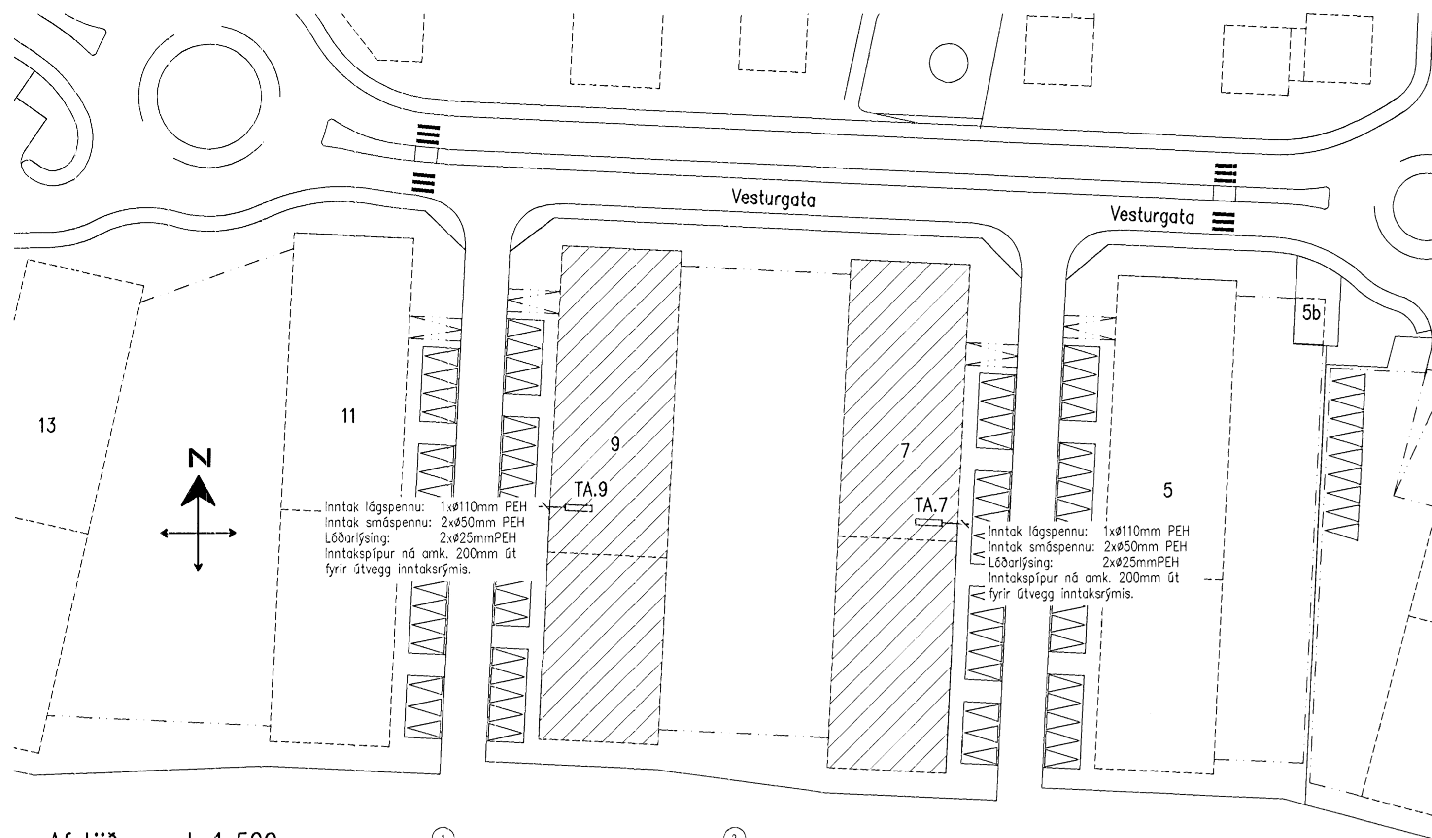
Afstöðumynd, 1:500
