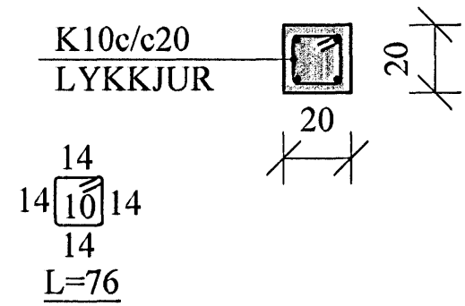
A13 I-13 SNIÐ. 1:20
