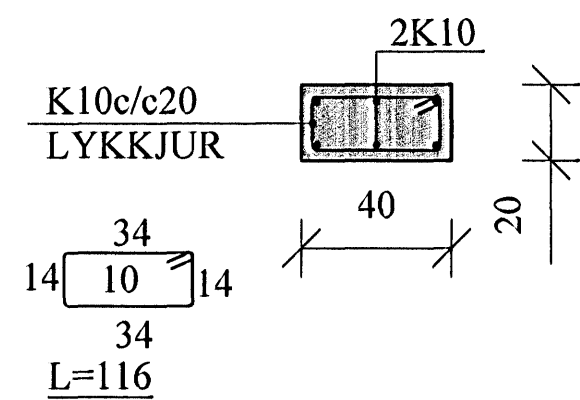
B13 I-13 SNIÐ. 1:20
