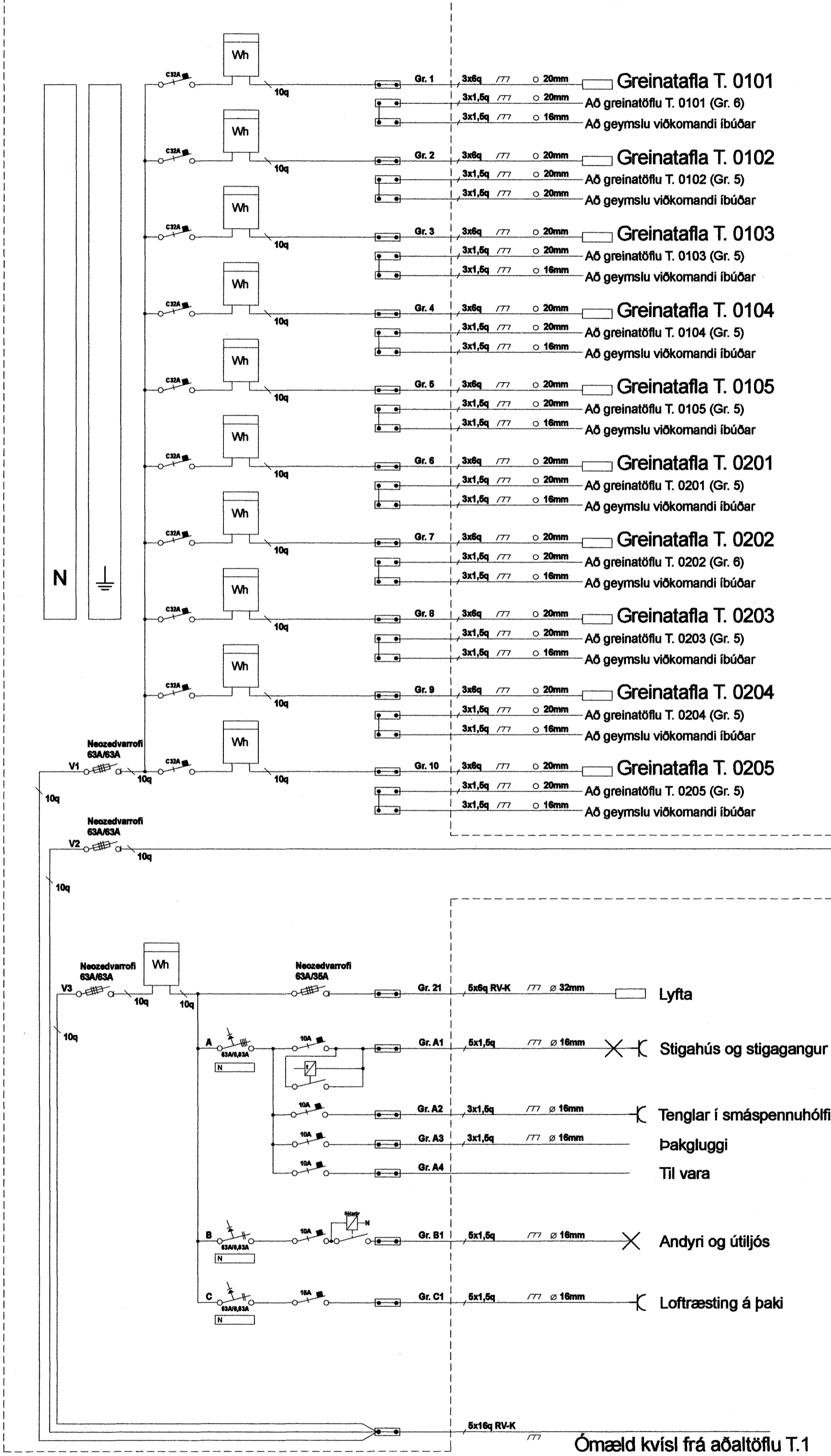
Einlínunmynd Töflu T.1.1 3/N ~ 400/230V
