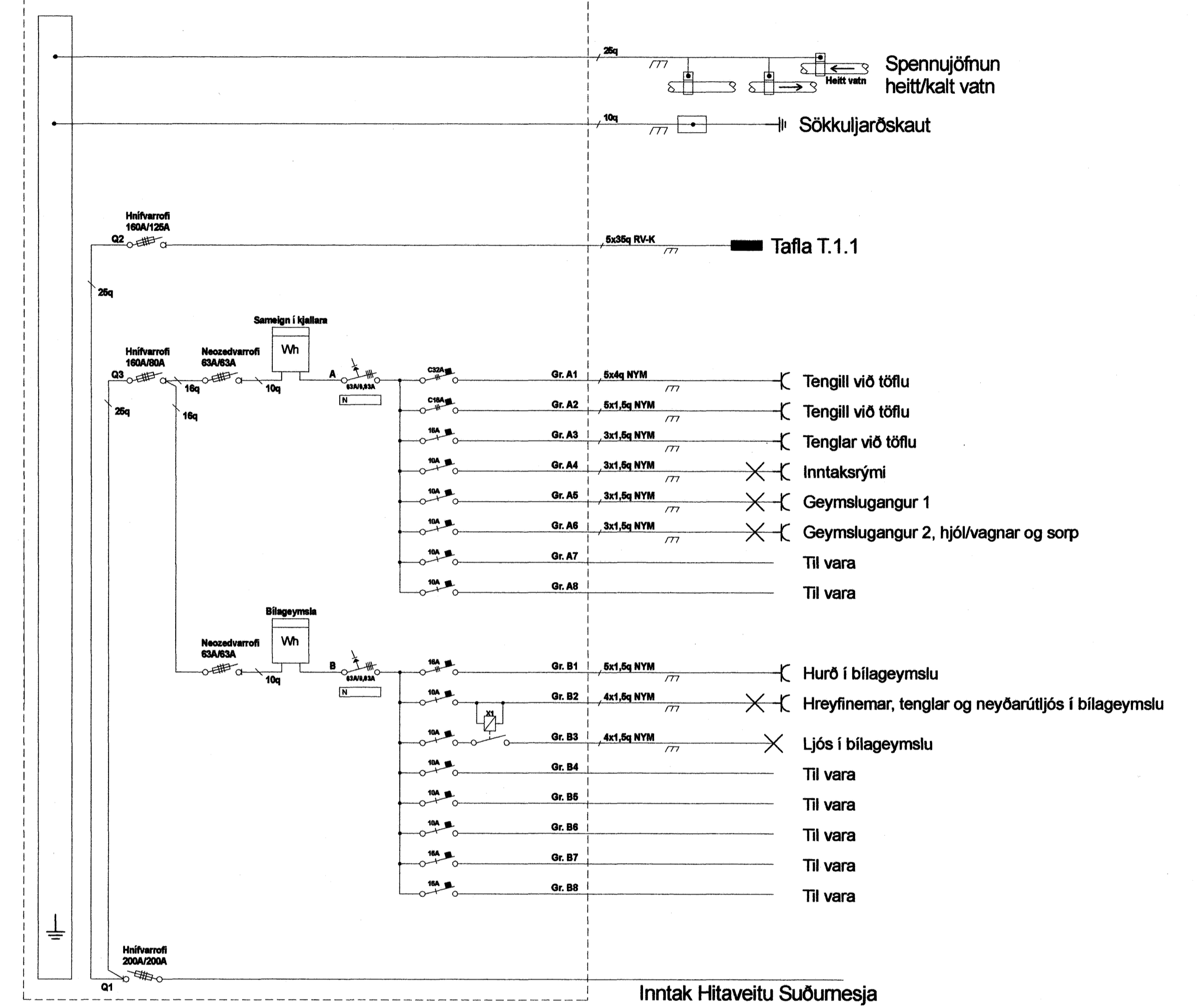
Einlínunmynd Töflu T.1 3/N ~ 400/230V
