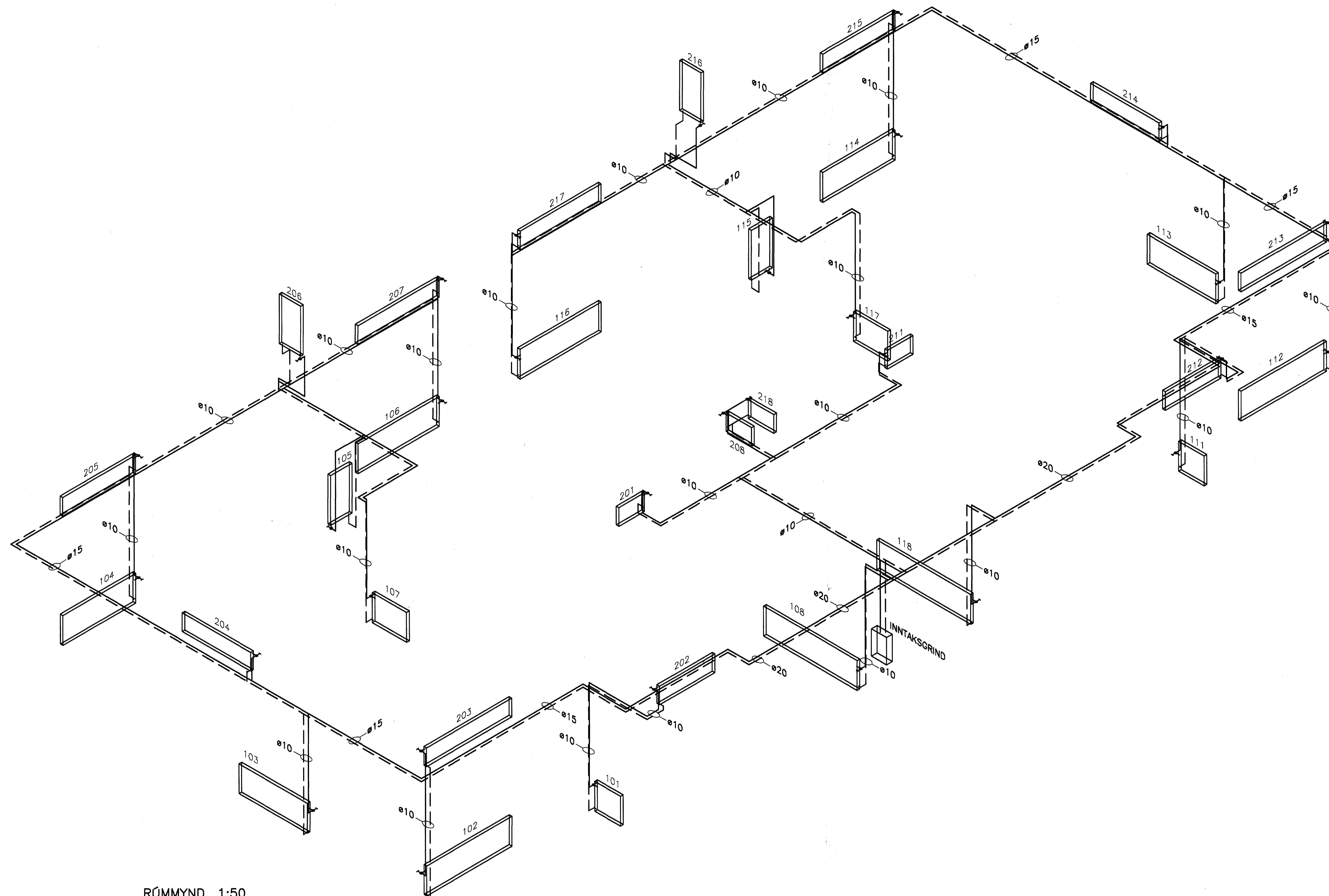
RÚMMYND. 1:50
