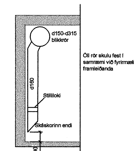
Frágangur útsogsstúta í bílakjallara
